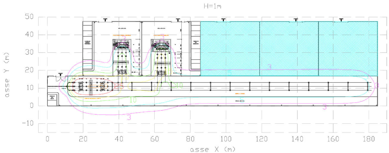
Figura 7 – Calcolo dei livelli di campo magnetico a 1 m da terra
