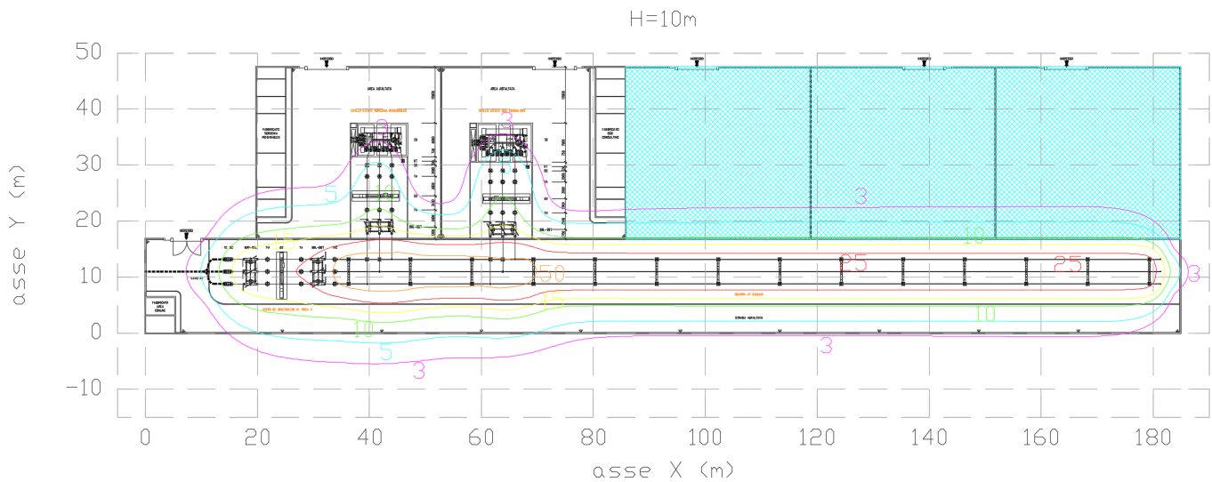
Figura 9 – Calcolo dei livelli di campo magnetico a 10 m da terra
