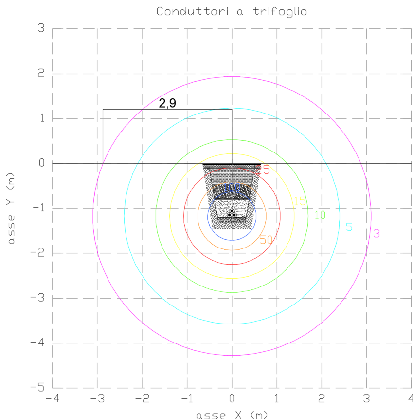
Figura 10 – Grafico dei livelli di campo magnetico prodotti dal cavidotto AT di connessione tra il Punto di Raccolta e la SE 380/150/36 kV Troia 2
