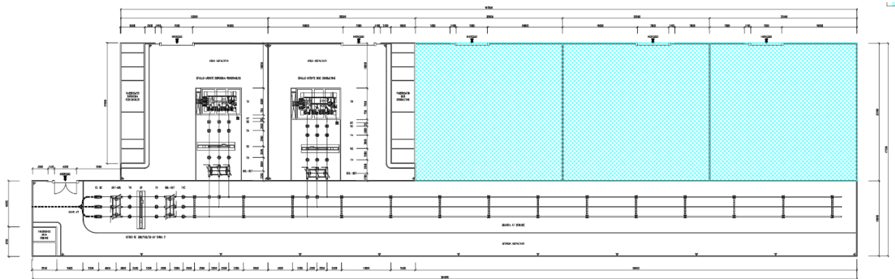
Figura 2: planimetria del Punto di Raccolta 150 kV "Masseria San Spirito"
