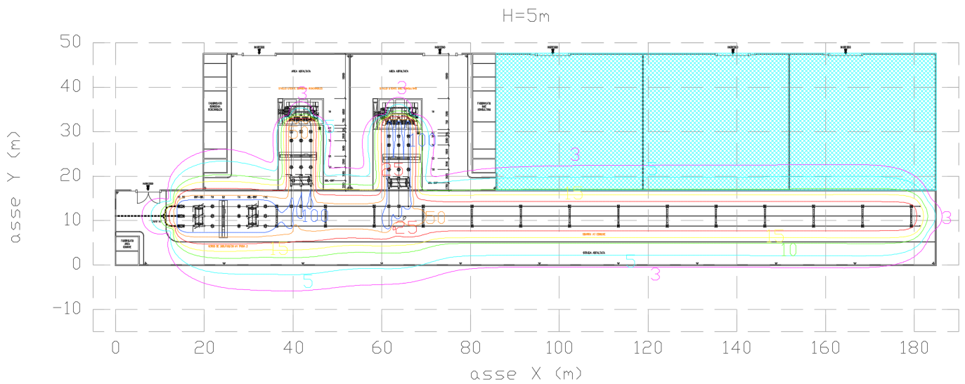
Figura 8 – Calcolo dei livelli di campo magnetico a 5 m da terra
