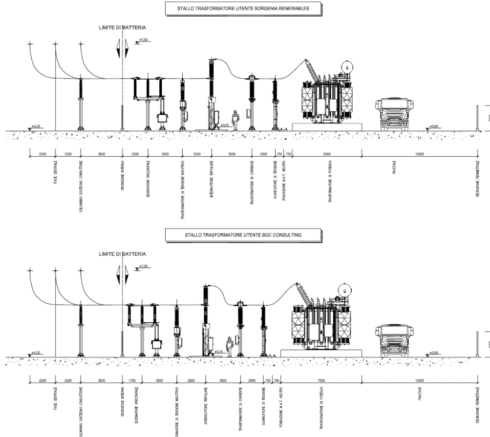
Figura 5 – Sezione dell'area utenti punto di raccolta 150 kV “Masseria San Spirito” con individuazione delle altezze
