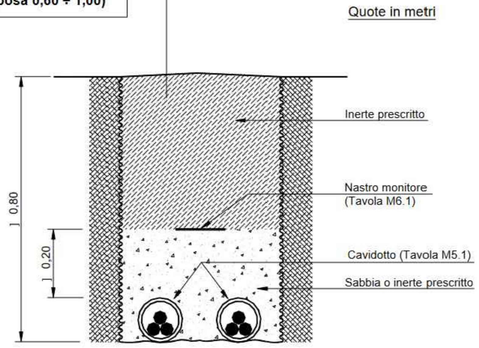
Canalizzazione Tipo A (profondità di posa 0,60 ± 1,00)
