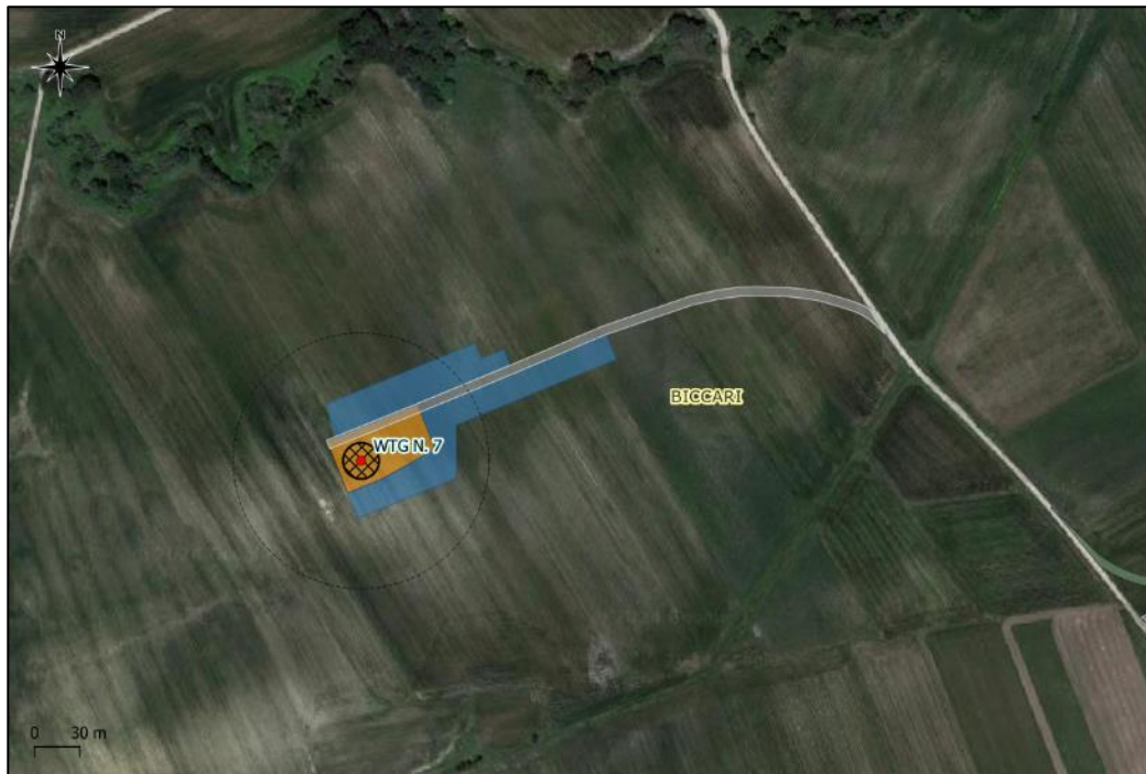
WTG 7 – Piazzola temporanea (in blu), permanente (in arancione) e viabilità di accesso (in grigio)
