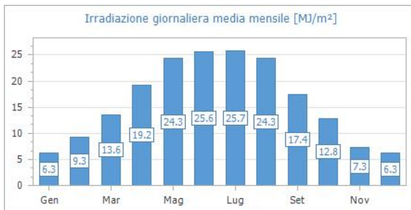
Fig. 1: Irradiazione giornaliera media mensile sul piano orizzontale [MJ/m²]- Fonte dati: UNI 10349:2016 - Stazione di rilevazione: Oppido Lucano
