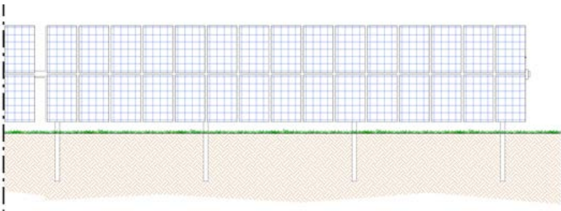
Figura 1 - dettaglio tracker
