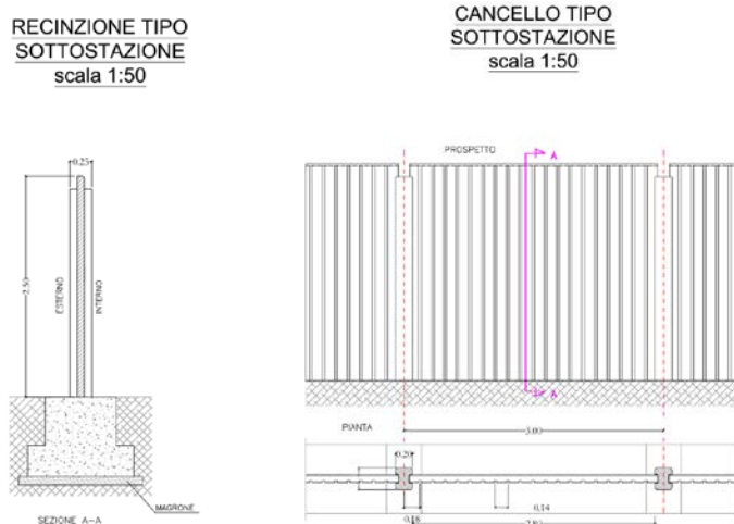
Figura 8 - Sezioni tipo recinzione e cancello SSE
