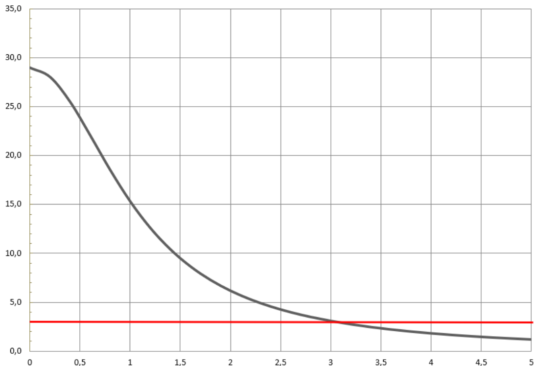
Figura 3 - Valore dell'induzione magnetica al livello del suolo nel tratto composto da n° 2 terne AT
