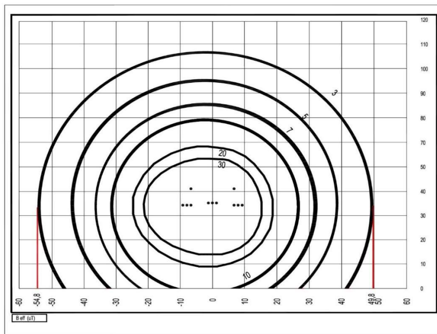
Figura 3: Curve di isocampo a 3 \mu\text{T} in una sezione perpendicolare all'asse linea per un sostegno in amarro 380 kV. DPA = 54,80m.
