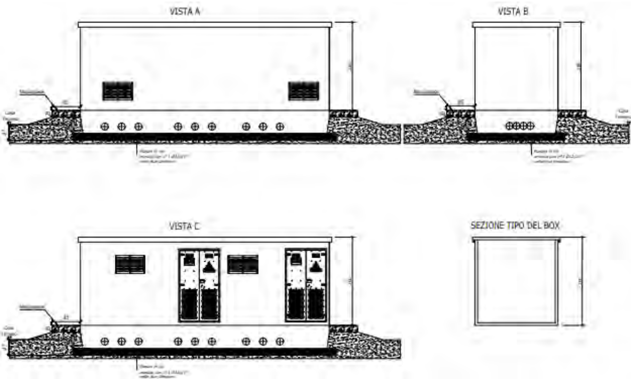
Figura 5.18 Vista cabine
