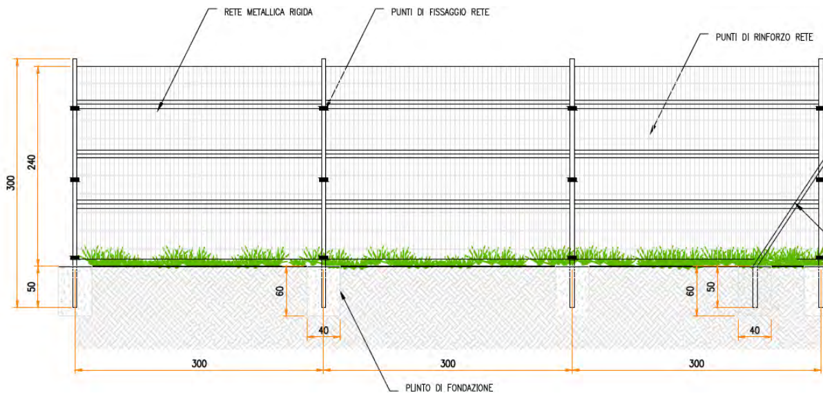
Figura 5.19 Tipologico recinzione perimetrale
