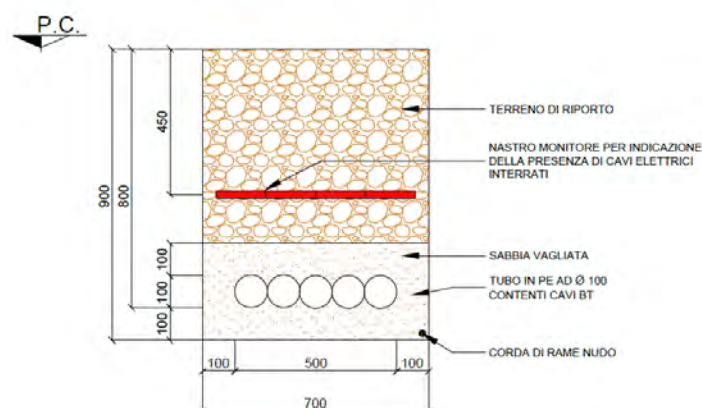
Figura 5.16: Sezione tipiche cavidotti interrati
