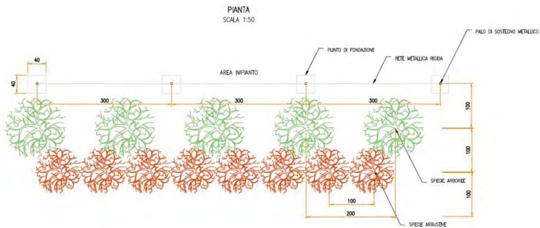
Figura 6.8 Tipologico del filare di mitigazione
