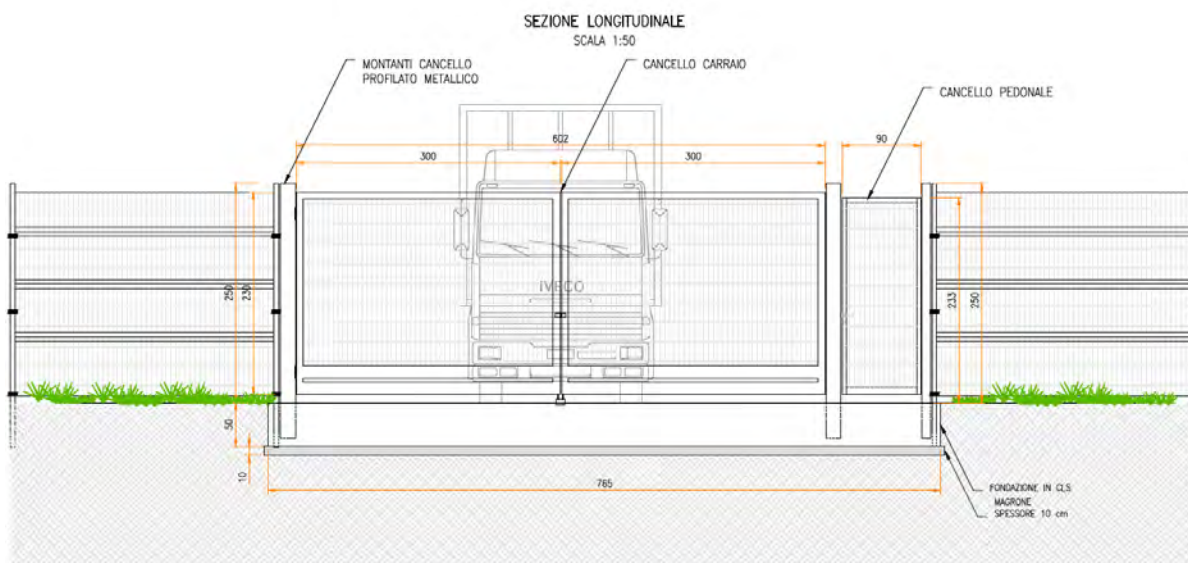
Figura 5.20 Tipologico cancelli accesso
