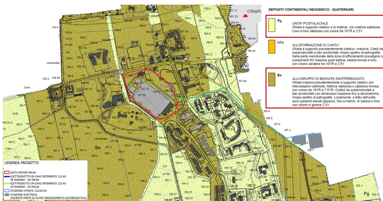
Figura 5-2: Stralcio Carta Geologica del Comune di Peschiera Borromeo (Fonte: Variante generale al Piano di Governo Del Territorio in attuazione alla L.R. 11/03/2005,n. 12 - AGGIORNAMENTO DELLA COMPONENTE GEOLOGICA, IDROGEOLOGICA E SISMICA ai sensi D.G.R. IX/2616 del 30/11/2011 e s.m.i - Maggio 2020)
