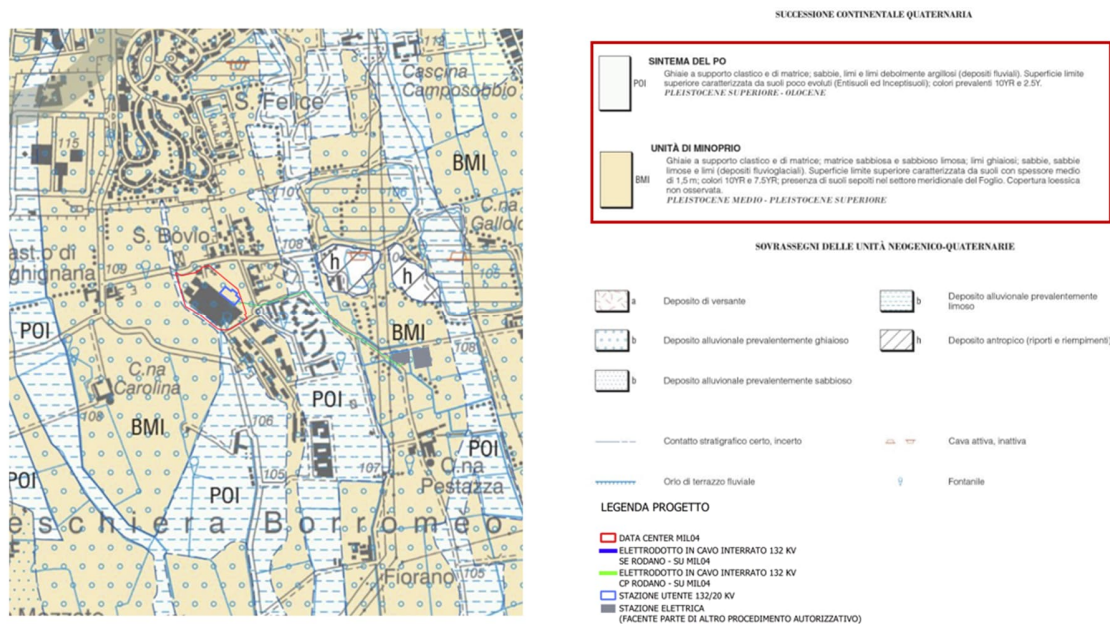
Figura 5-1: Stralcio della Carta Geologica 1:50.000 (Foglio 118 Milano. Fonte: 118 Milano (ispambiente.gov.it) )
