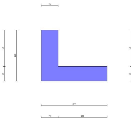
Fig. 1 - Sezione quotata del muro
