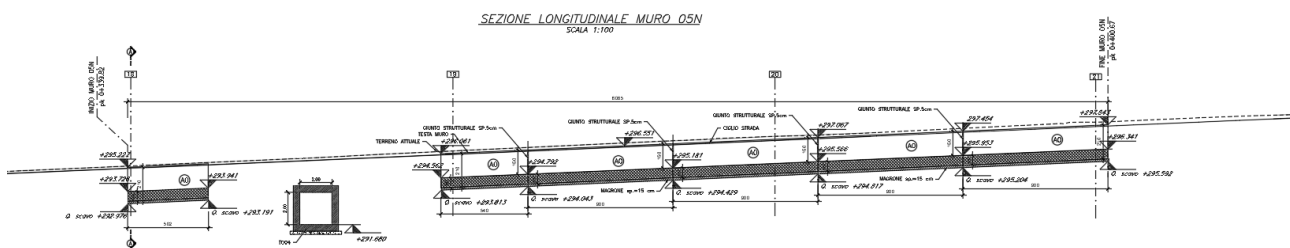
Figura 3: profilo longitudinale
