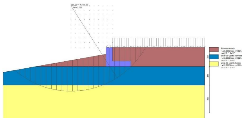
Fig. 10 - Stabilità fronte di scavo - Cerchio critico (Combinazione n° 2)
