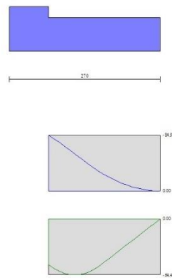
Fig. 12 - Fondazione
