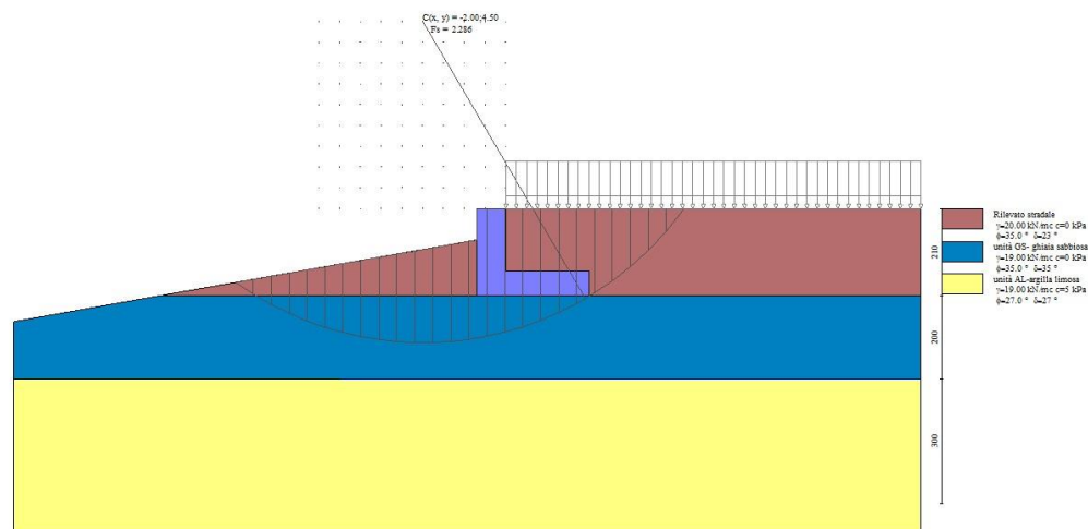
Figura 20: Stabilità fronte di scavo - Cerchio critico (Combinazione n° 4)_FS=2.286
