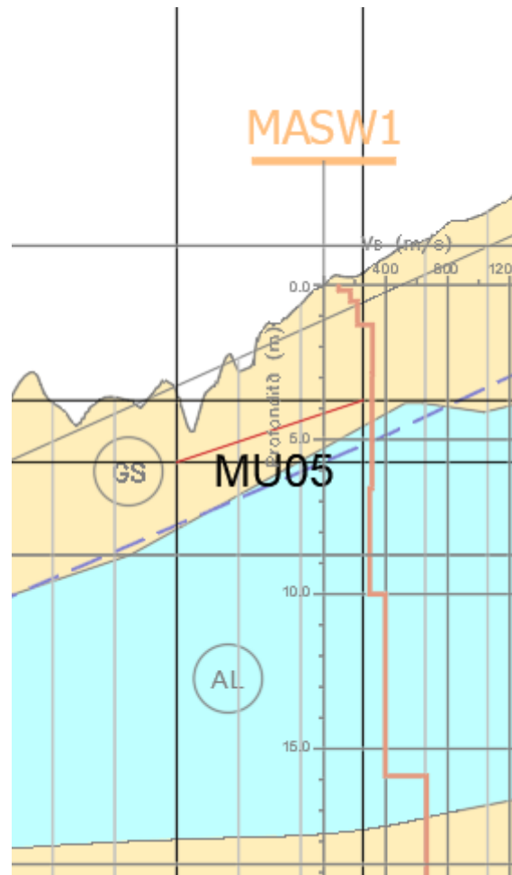
Figura 5: Stralcio del profilo geotecnico con ubicazione dell'opera
