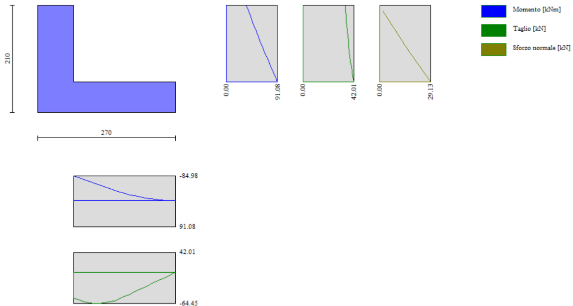
Figura 19: Inviluppo diagrammi sollecitazioni – condizione urto
