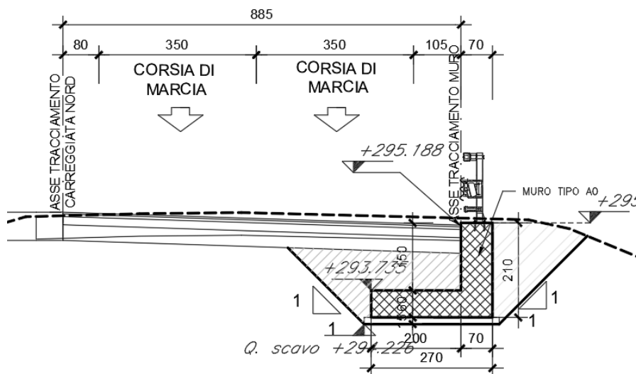
Figura 4: sezione trasversale muro tipologico A0
