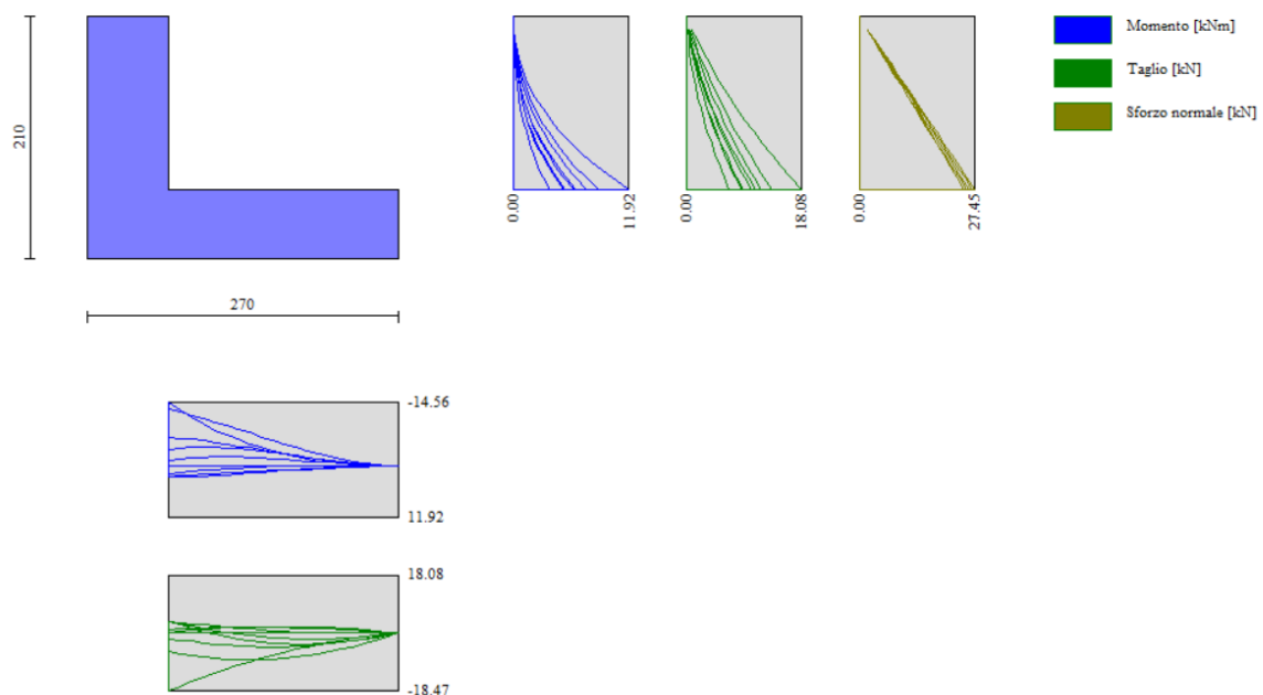
Figura 18: Involuppo diagrammi sollecitazioni- condizioni statiche e sismiche
