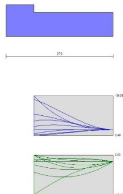
Fig. 16 - Fondazione
