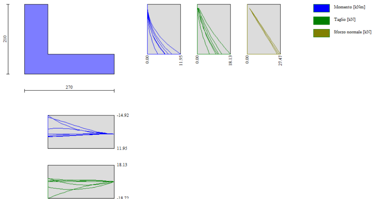
Figura 18: Inviluppo diagrammi sollecitazioni- condizioni statiche e sismiche
