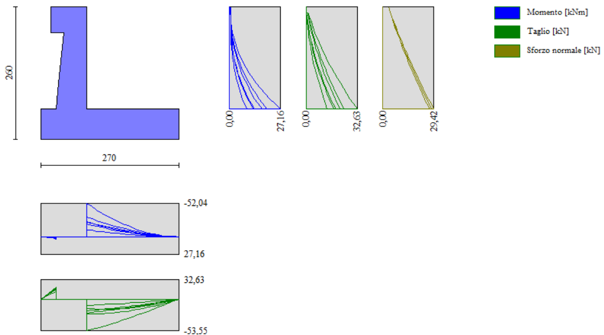
Figura 27: Involuppo diagrammi sollecitazioni- condizioni statiche e sismiche
