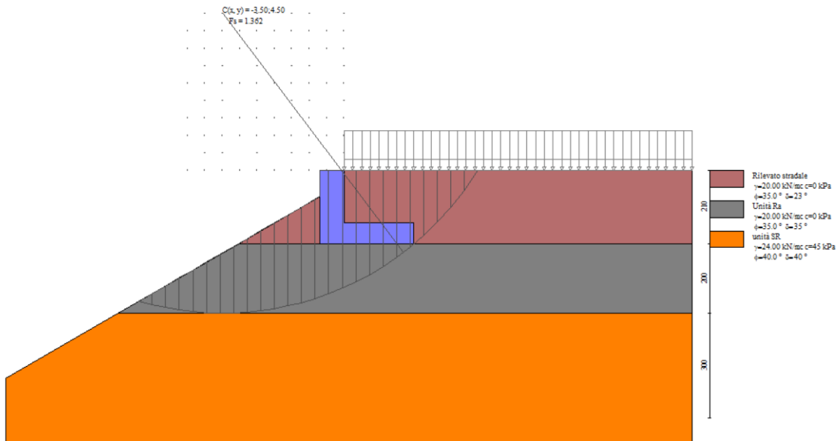
Figura 20: Stabilità fronte di scavo - Cerchio critico (Combinazione n° 4)_FS=1.362
