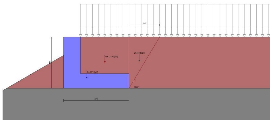
Fig. 3 - Cuneo di spinta (combinazione statica) (Combinazione n° 1)
