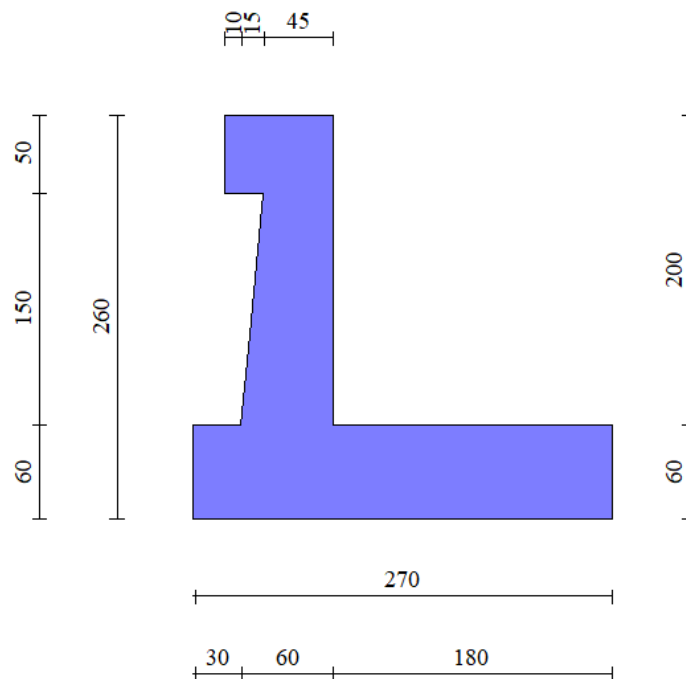
Figura 23: modello di calcolo muro tipologico A
