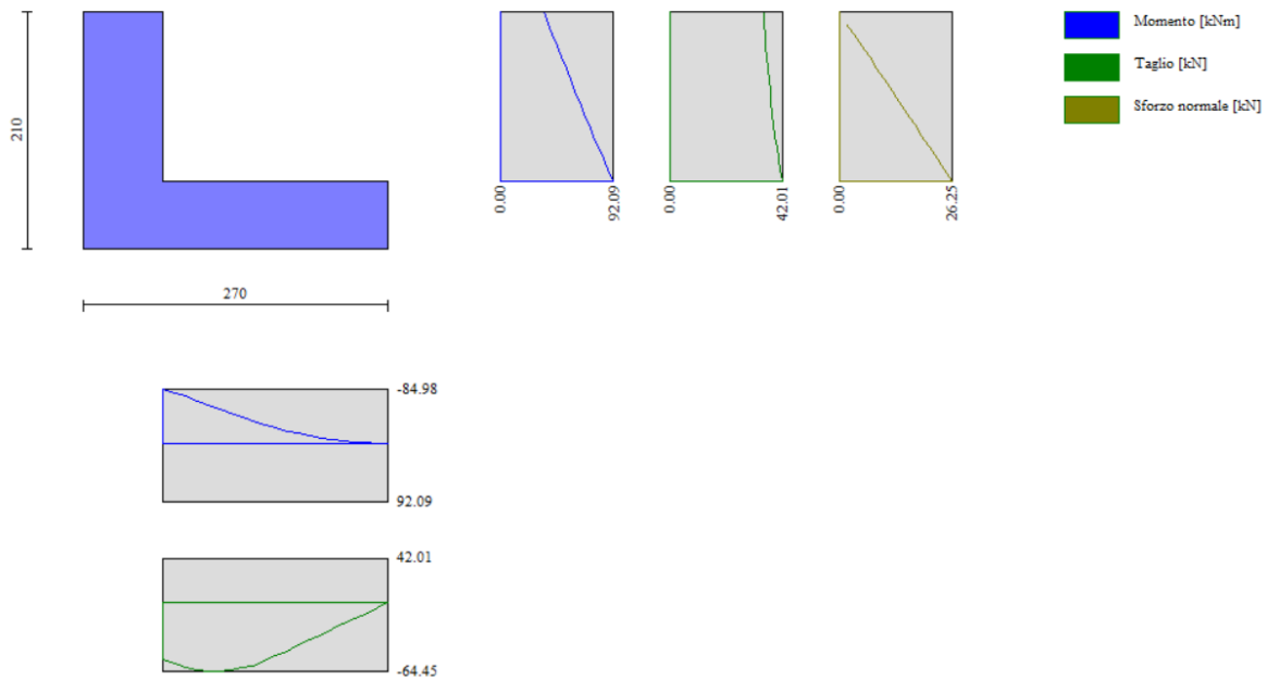
Figura 19: Involuppo diagrammi sollecitazioni – condizione urto
