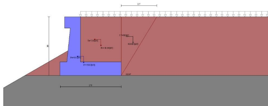
Fig. 5 - Cuneo di spinta (combinazione sismica) (Combinazione n° 2)
