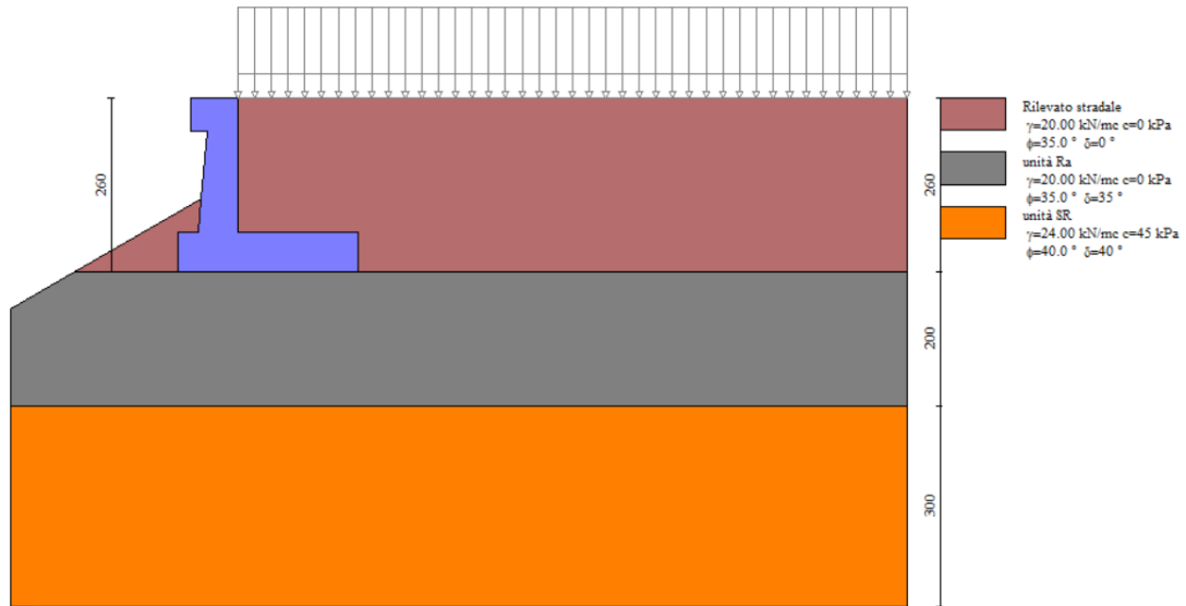
Figura 23: modello di calcolo muro tipologico A
