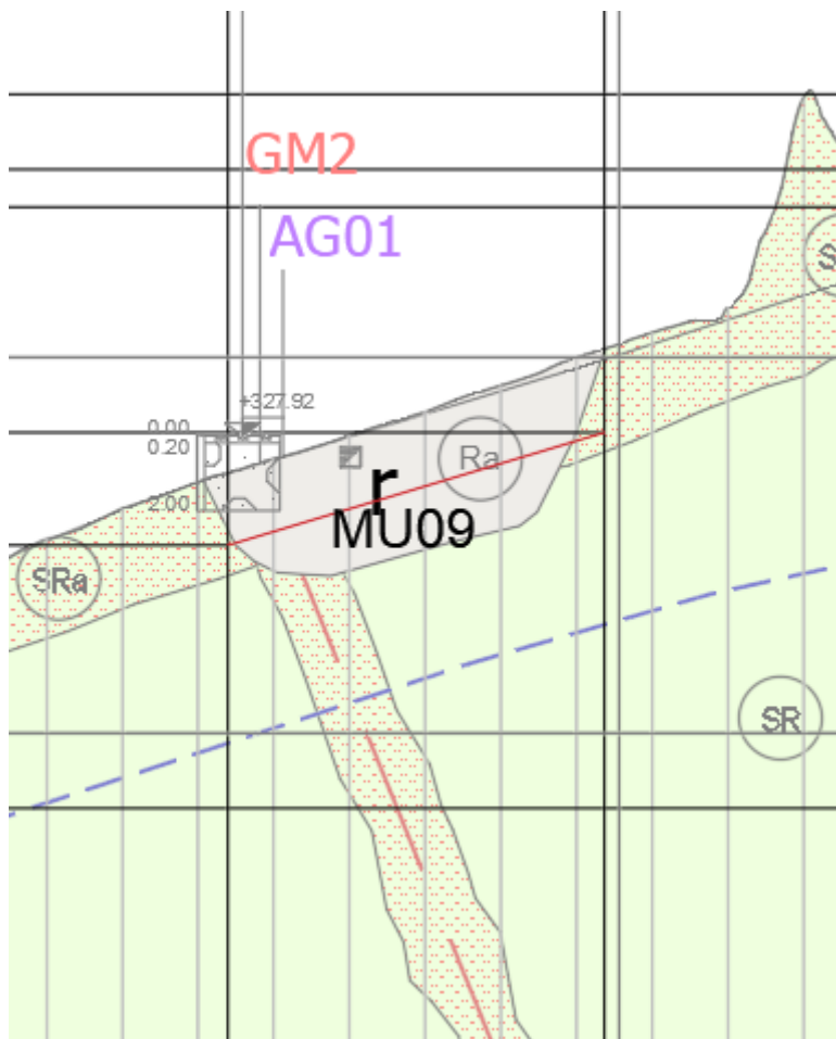
Figura 5: Stralcio profilo geotecnico con ubicazione dell'opera
