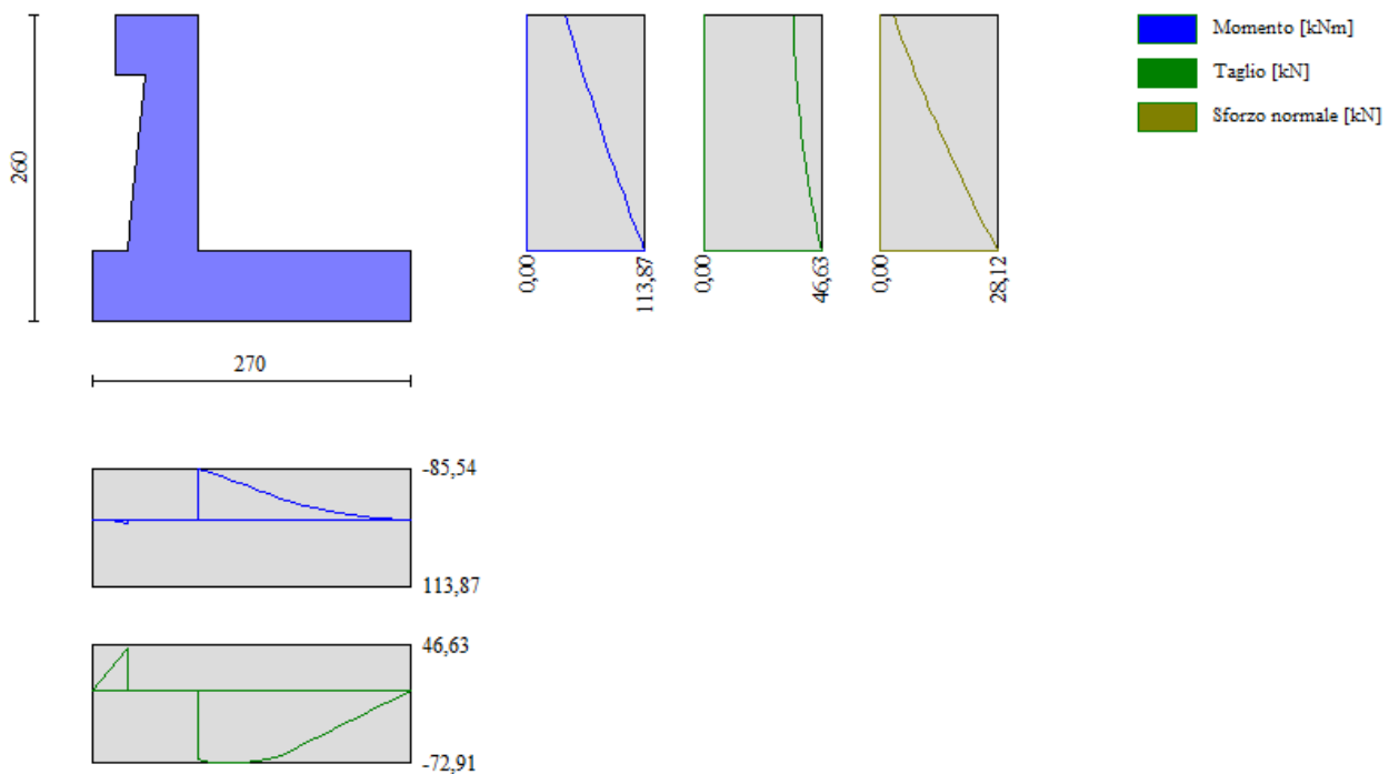
Figura 28: Involuppo diagrammi sollecitazioni – condizione urto
