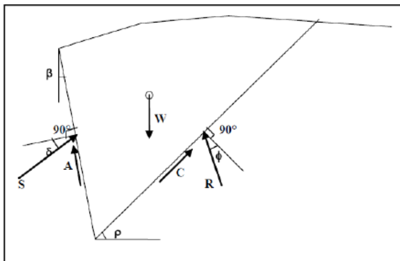
Figura 13: schema metodo di Culmann per calcolo della spinta
