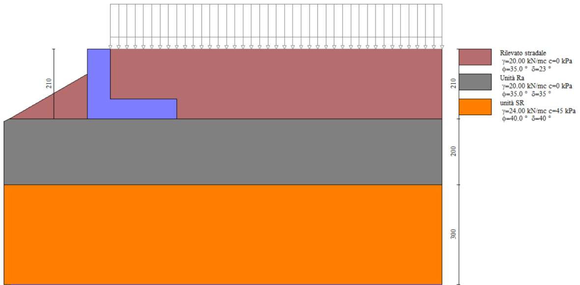
Figura 14: modello di calcolo muro tipologico A0
