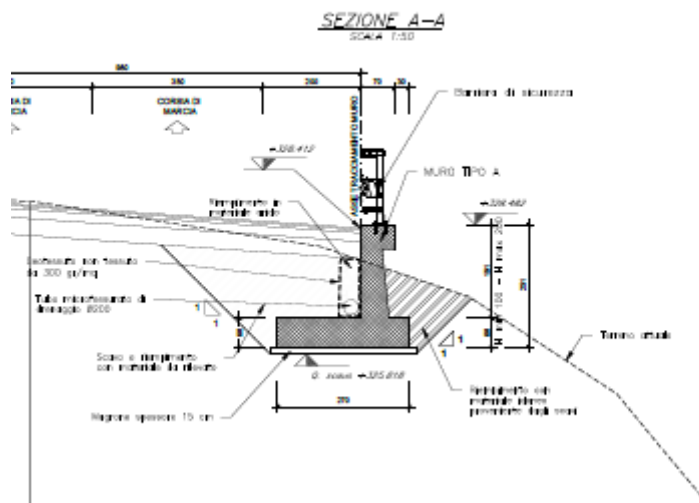
Figura 4: sezione trasversale muro tipologico A
