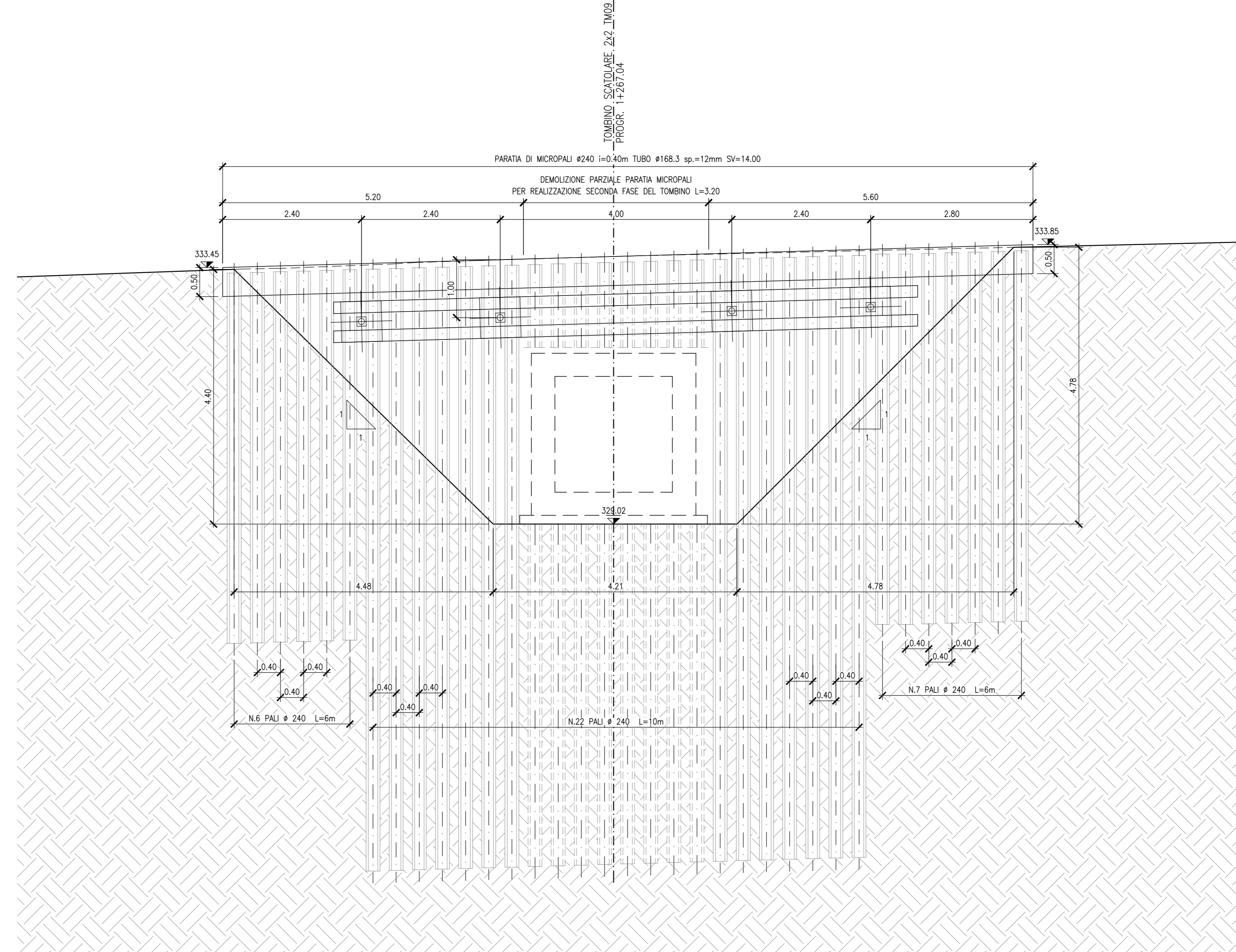
SEZIONE LONGITUDINALE B-B SECONDA FASE - Scala 1:50 -
