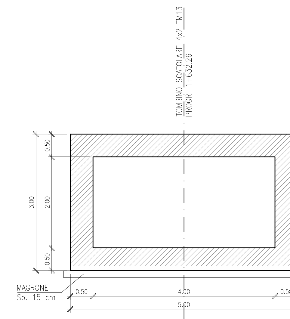
SEZIONE C-C - Scala 1:50 -
