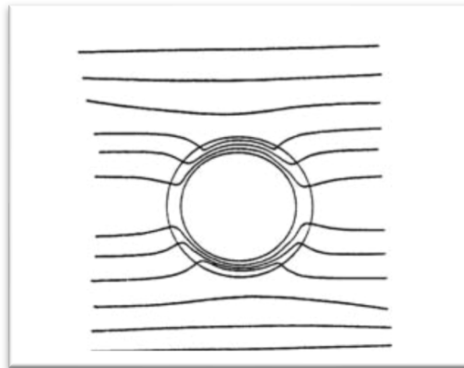
Figura 10: andamento qualitativo della deformazione delle linee di forza di un campo magnetico uniforme per effetto di un nucleo in materiale ferromagnetico
