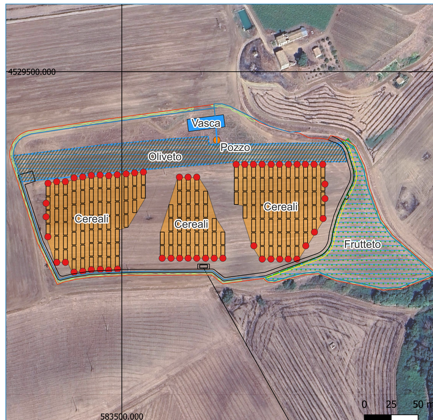
Impianto irriguo - Oliveto, Frutteto e siepe Mirto
