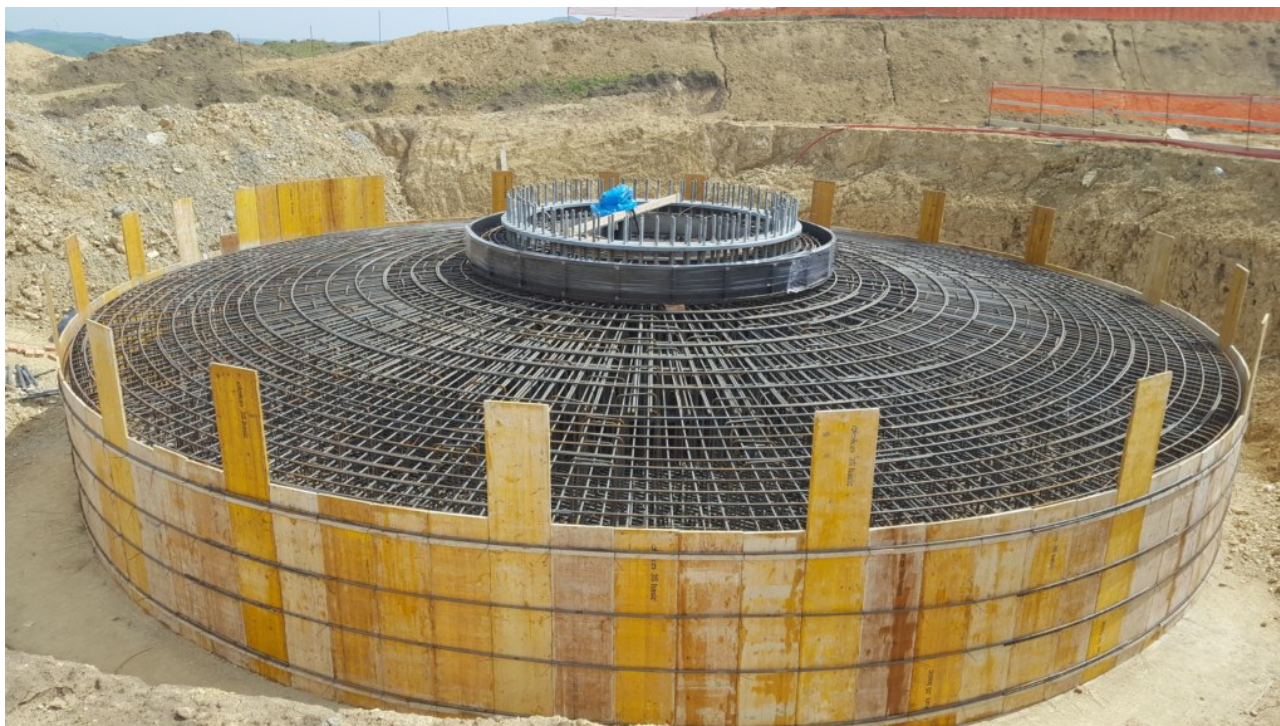
Figura 4 | Strutture di fondazione degli aerogeneratori
