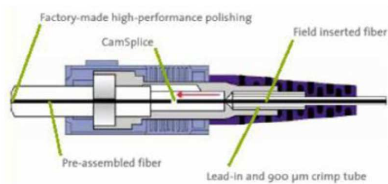
Figura 7 | Connettore ST
