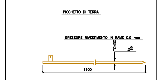
TIPICO PICCHETTI E CORDE DI TERRA
