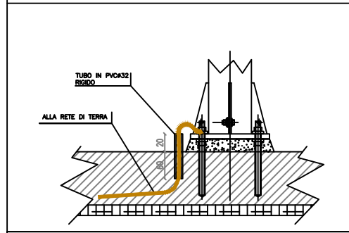
TIPICO MESSA A TERRA SOSTEGNO METALLICO
