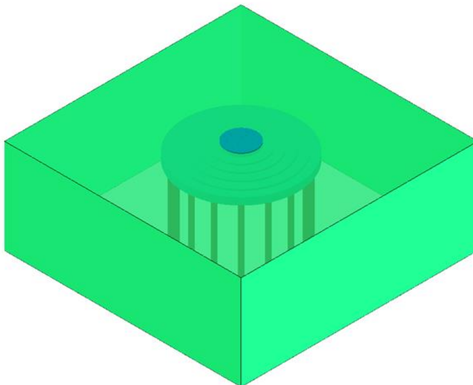
Figura 4 - Modellazione fondazione e stratigrafia
