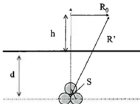
Figura 14 - Schema di principio per il calcolo delle distanze da terne di cavi interrati con poa a trifoglio oltre le quali l'induzione magnetica è inferiore all'obiettivo i qualità
