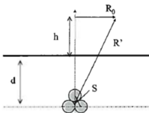
Figura 15 - Schema di principio per il calcolo delle distanze da terne di cavi interrati con posa a trifoglio oltre le quali l'induzione magnetica è inferiore all'obiettivo i qualità
