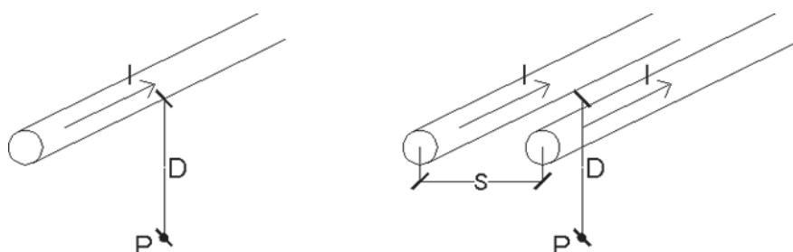
Figura 10 - Linea Unifilare e Bifilare
