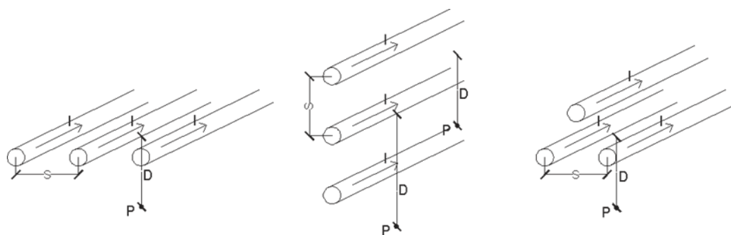
Figura 11 - Schemi dei sistemi trifase (conduttori in piano, in verticale, a triangolo)
