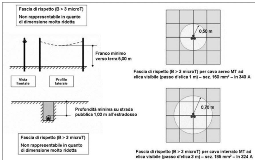
Figura 8 - Fasce di rispetto DPA
