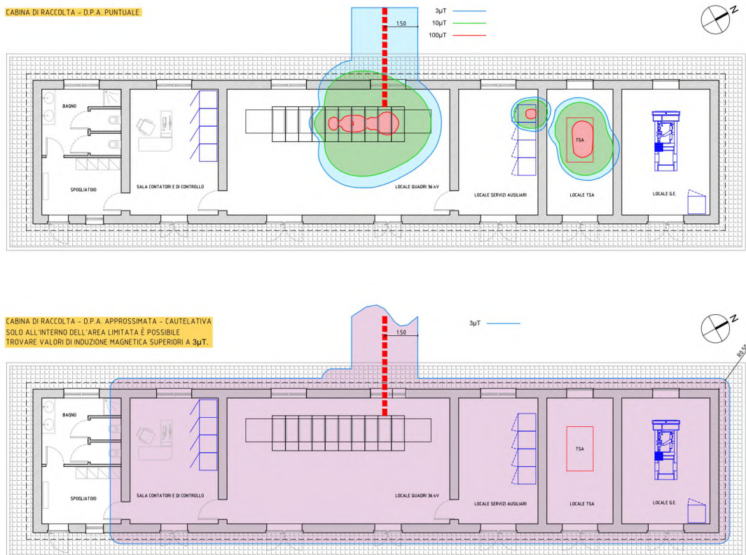
Figura 5 - Cabina di Raccolta e Trasmissione calcolo puntuale ed approssimazione cautelativa
