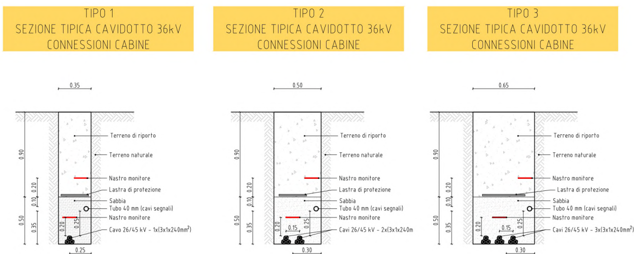
Figura 1 - Vista in sezione di una due o tre terne interrate.
