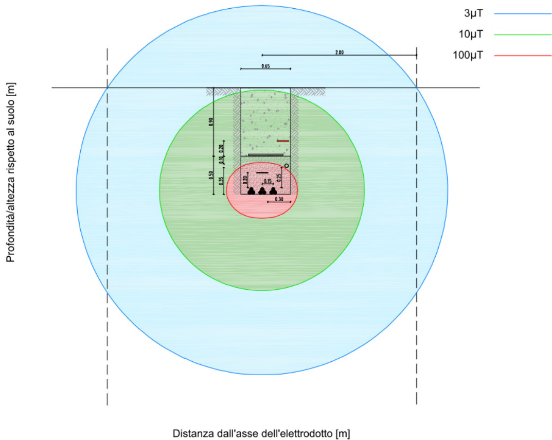
Figura 4 - Isolinee 3, 10 e 100 µT – Sezione con tre terne interrate - Tipo 3
