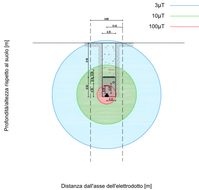
Figura 2 - Isolinee 3, 10 e 100 \mu T – Sezione con una terza interrata - Tipo 1
