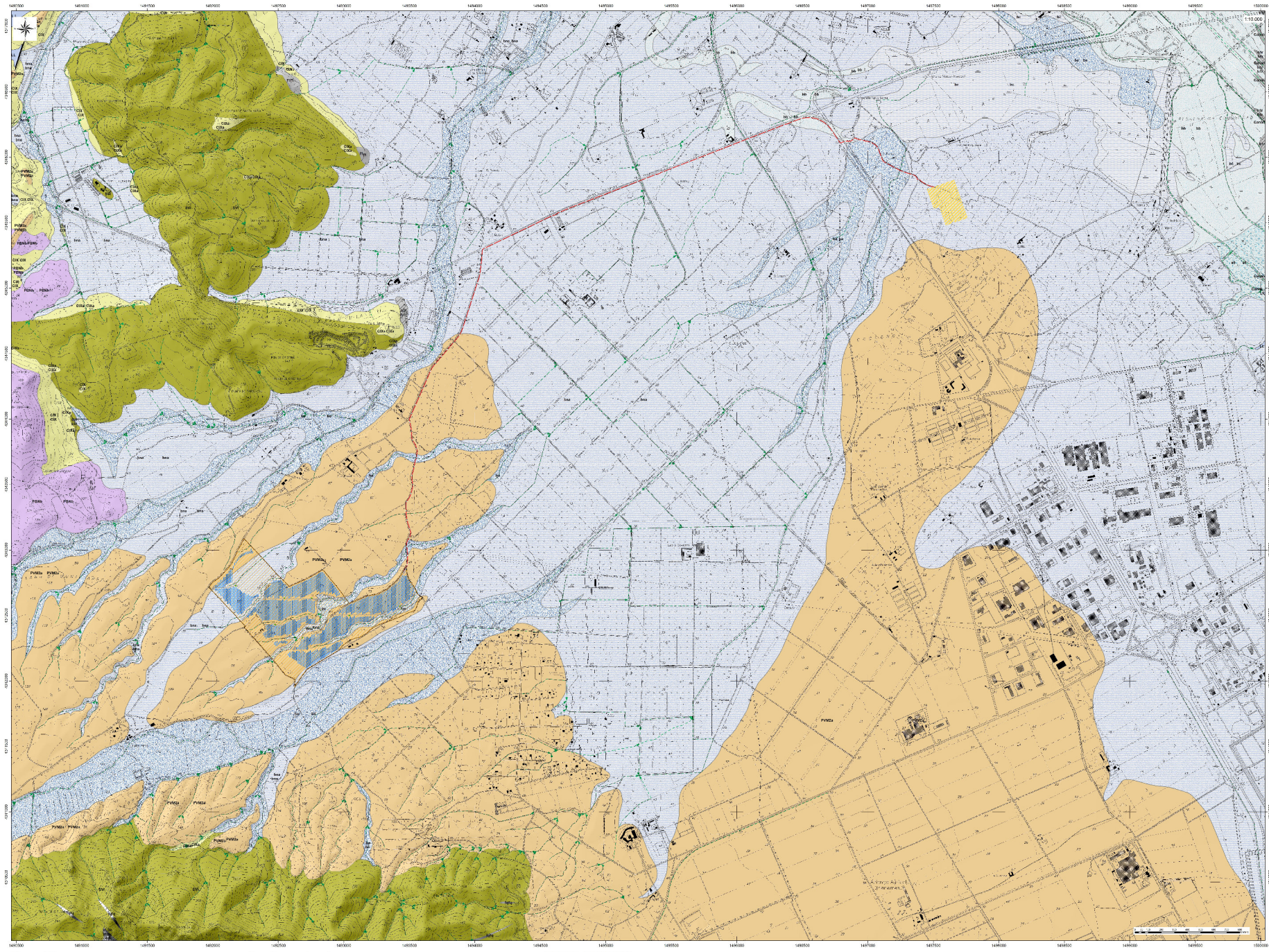
Stralcio della Carta Geomorfologica della Sardegna marina e continentale (A. Uzega, 1966)
