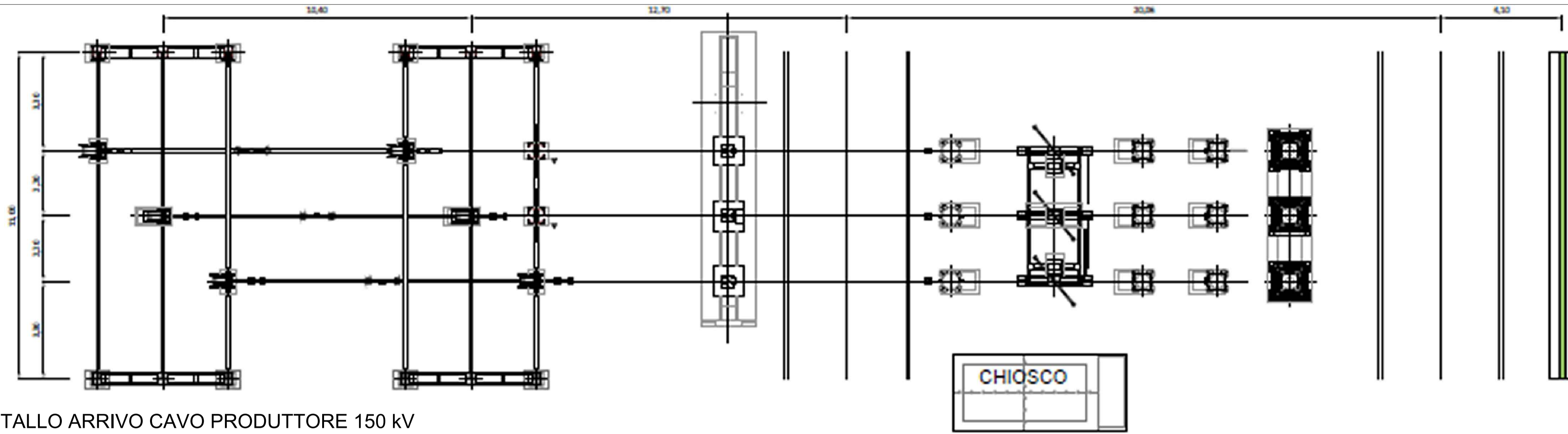
SEZIONE STALLO ARRIVO CAVO PRODUTTORE 150 KV
