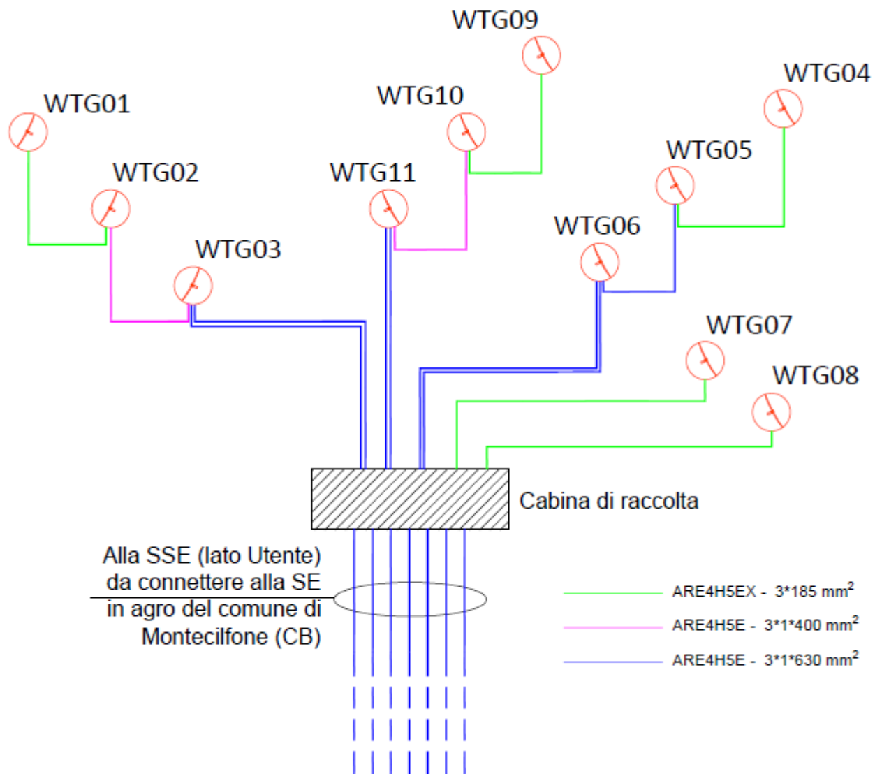
Figura 3 - Schema di connessione elettrica dell'impianto eolico in progetto
