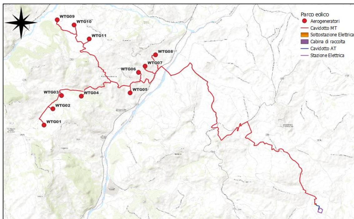
Figura 1 - Tavola di inquadramento su viabilità gruppo aerogeneratori WTG 01-11
