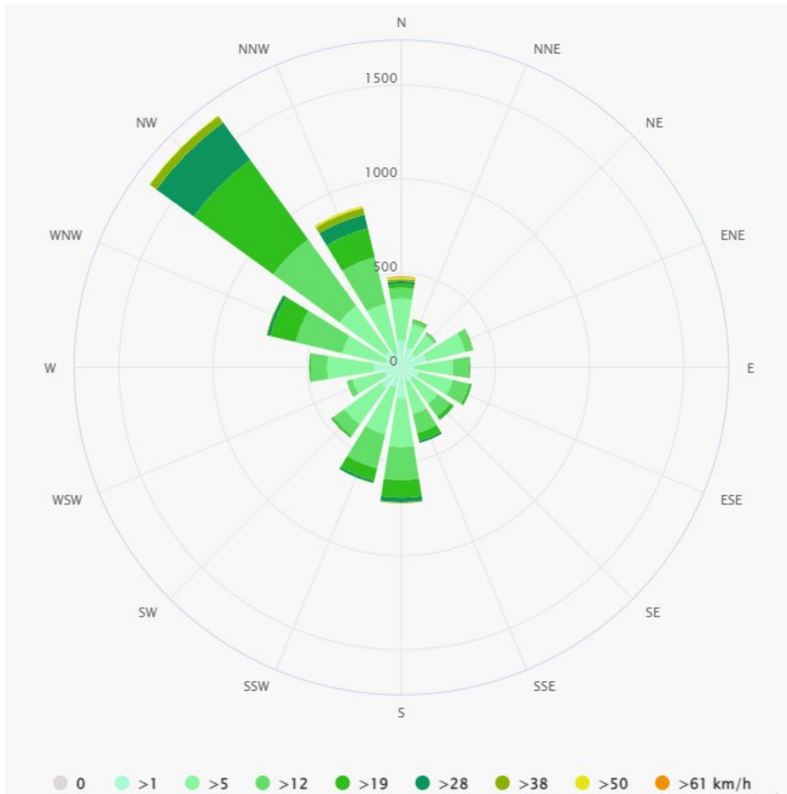
Fresagrandinaria, Dogliola e Lentella - Direzione prevalente del vento NO
