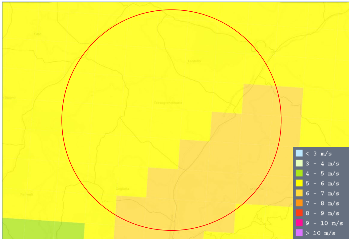
Figura 9 - Velocità del vento a 100 m s.l.t.
