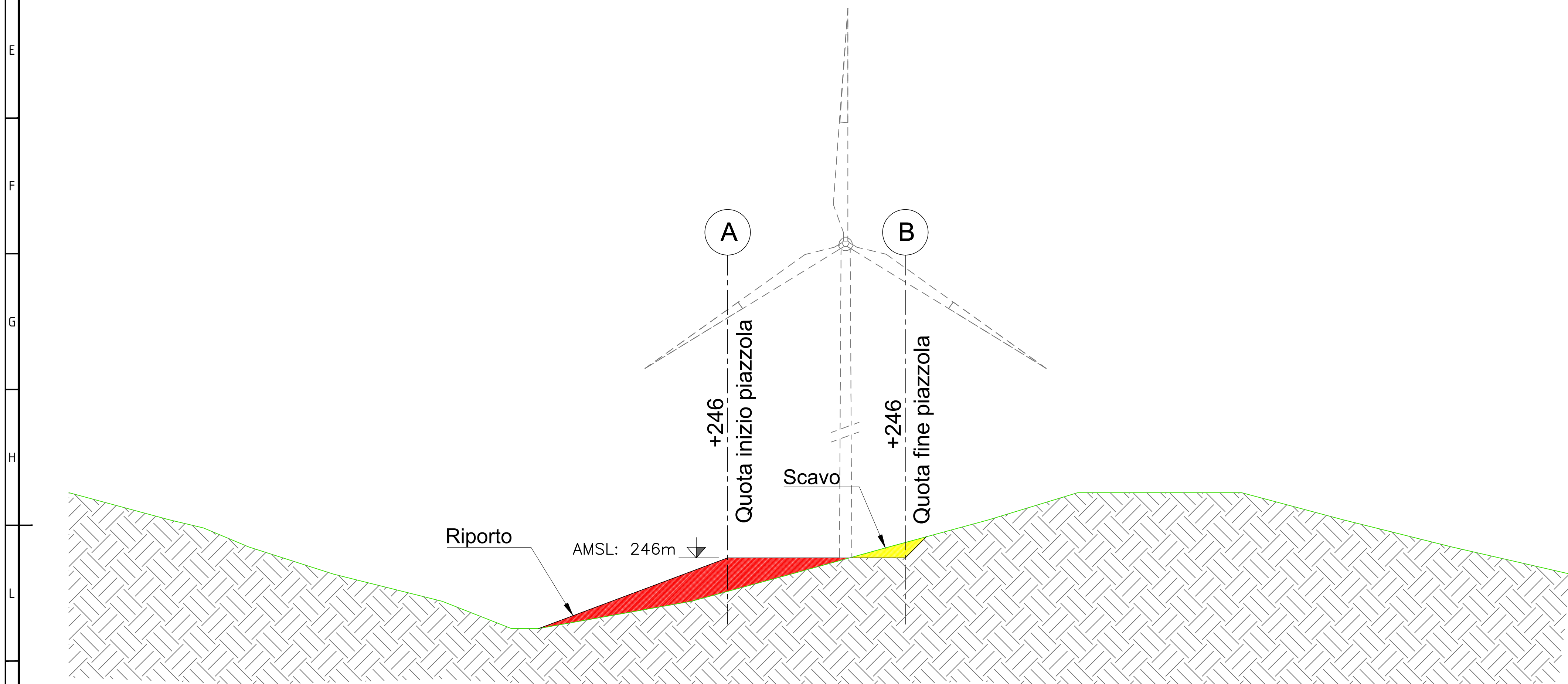
SEZIONE M-M- FASE DI CANTIERE scala 1:100
