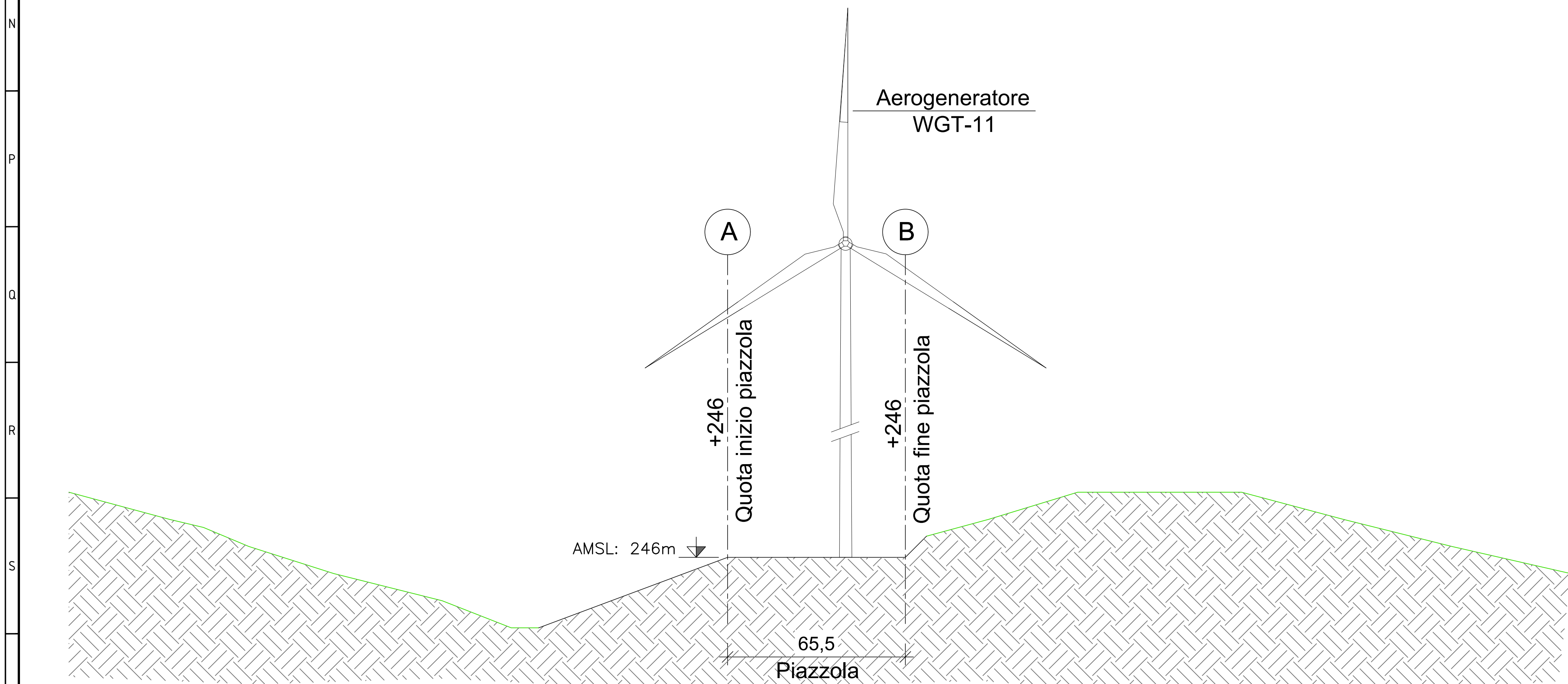
SEZIONE M-M- FASE DI ESERCIZIO scala 1:100
