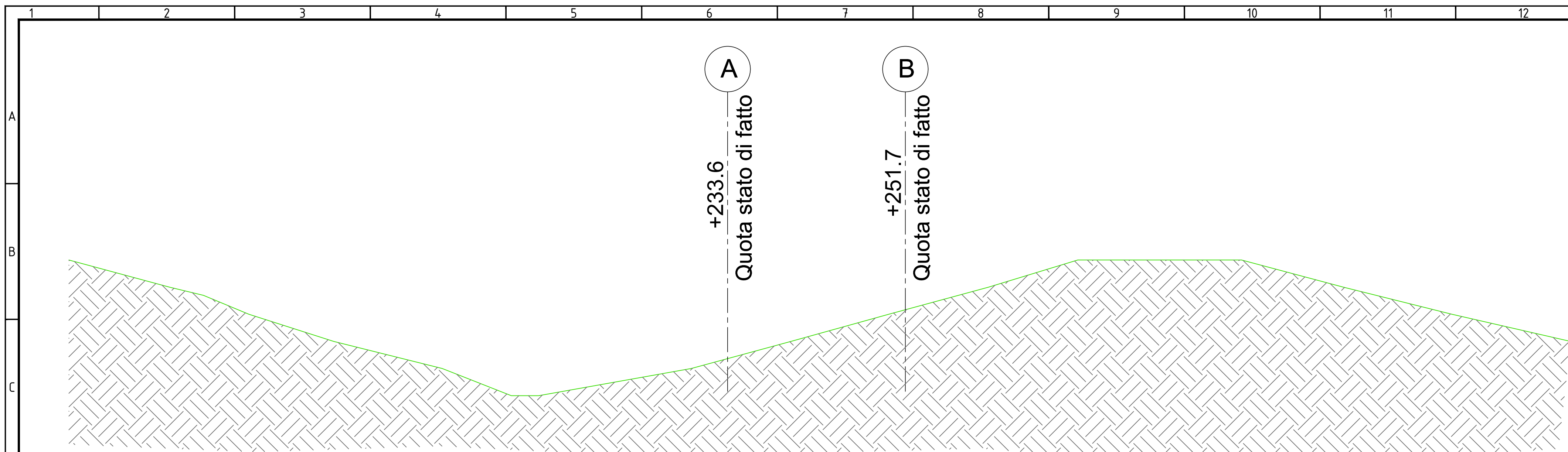
SEZIONE M-M - STATO DI FATTO scala 1:100
