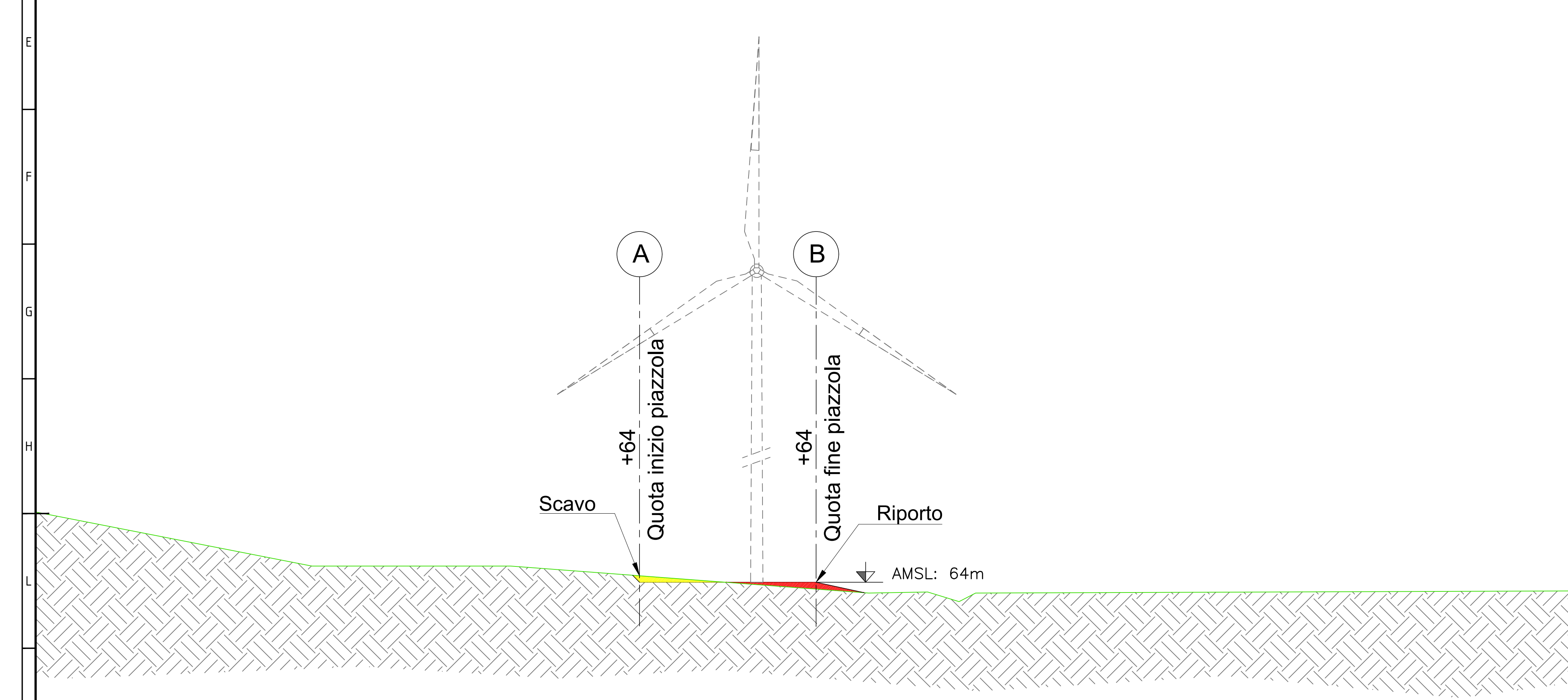
SEZIONE B-B - FASE DI CANTIERE scala 1:100
