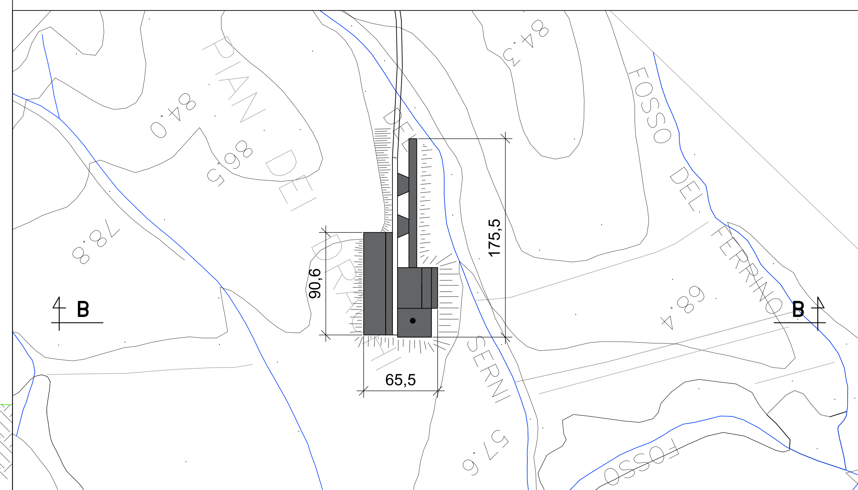
VISTA IN PIANTA PIAZZOLA WGT-2 FASE DI CANTIERE scala 1:200
