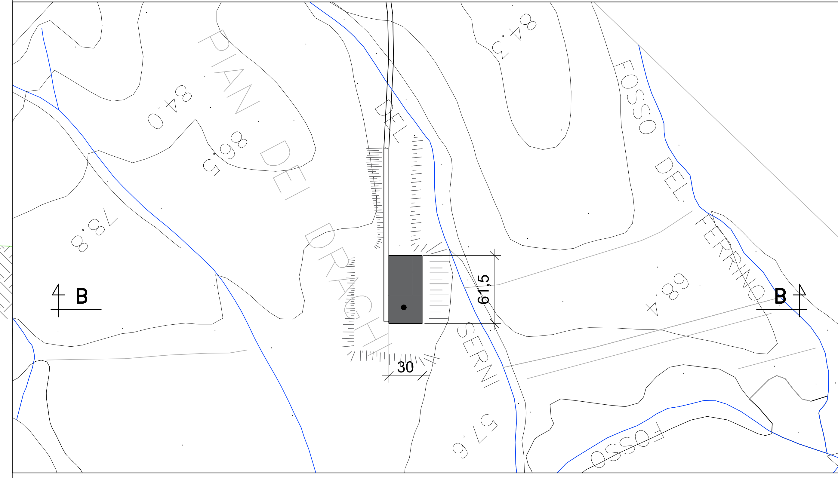
VISTA IN PIANTA PIAZZOLA WGT-2 FASE DI ESERCIZIO scala 1:200
