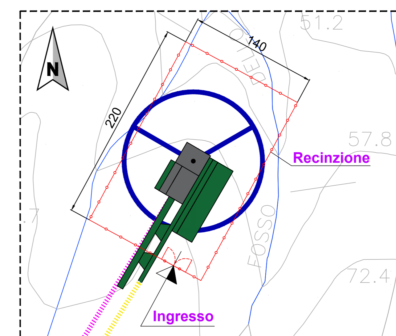
INQUADRAMENTO CANTIERE WTG1 (NON IN SCALA)
