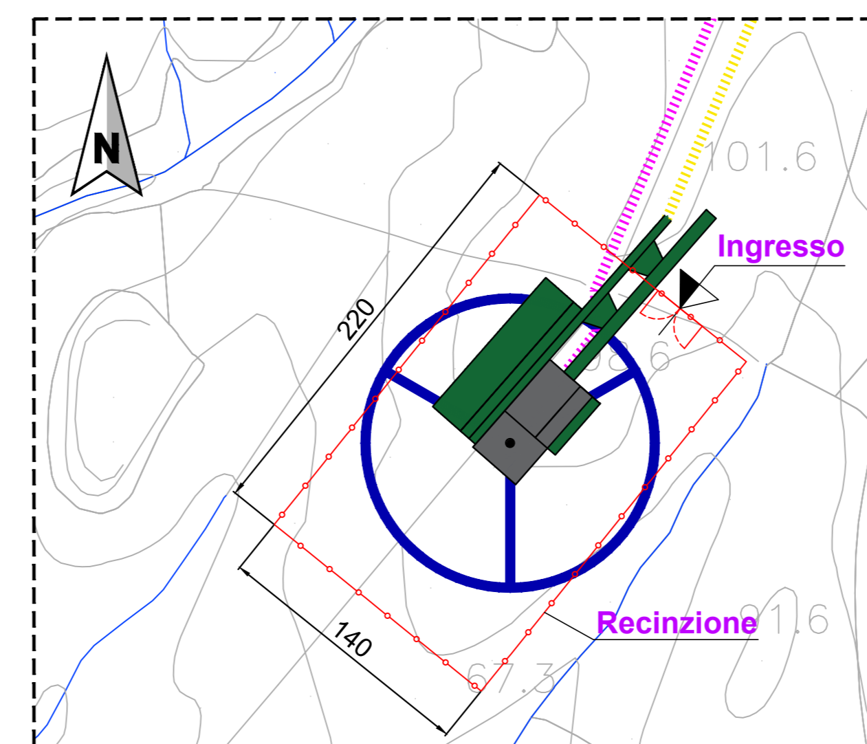
INQUADRAMENTO CANTIERE WTG3 (NON IN SCALA)
