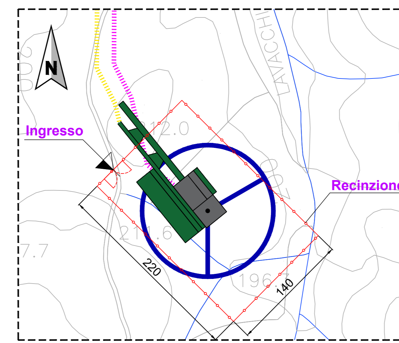
INQUADRAMENTO CANTIERE WTG8 (NON IN SCALA)
