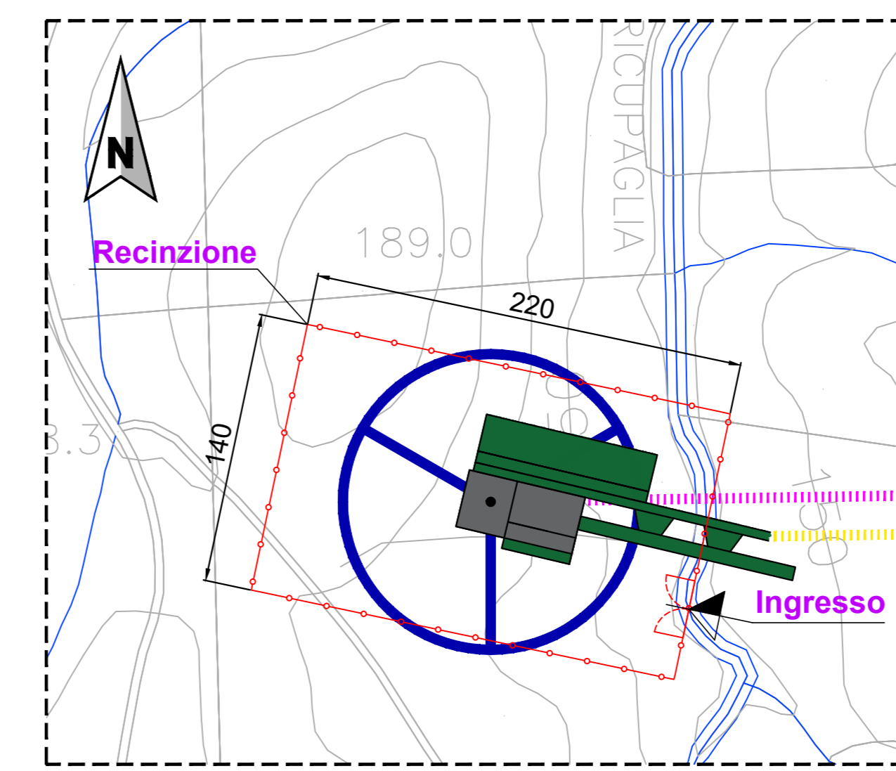
INQUADRAMENTO CANTIERE WTG9 (NON IN SCALA)
