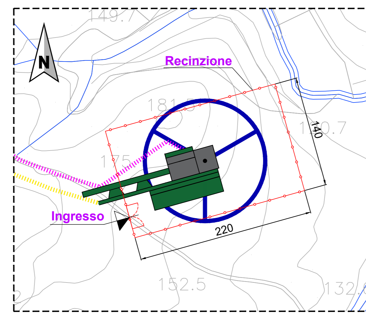
INQUADRAMENTO CANTIERE WTG7 (NON IN SCALA)
