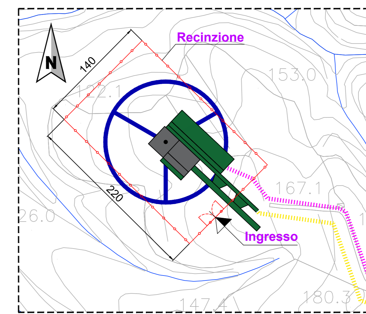
INQUADRAMENTO CANTIERE WTG6 (NON IN SCALA)
