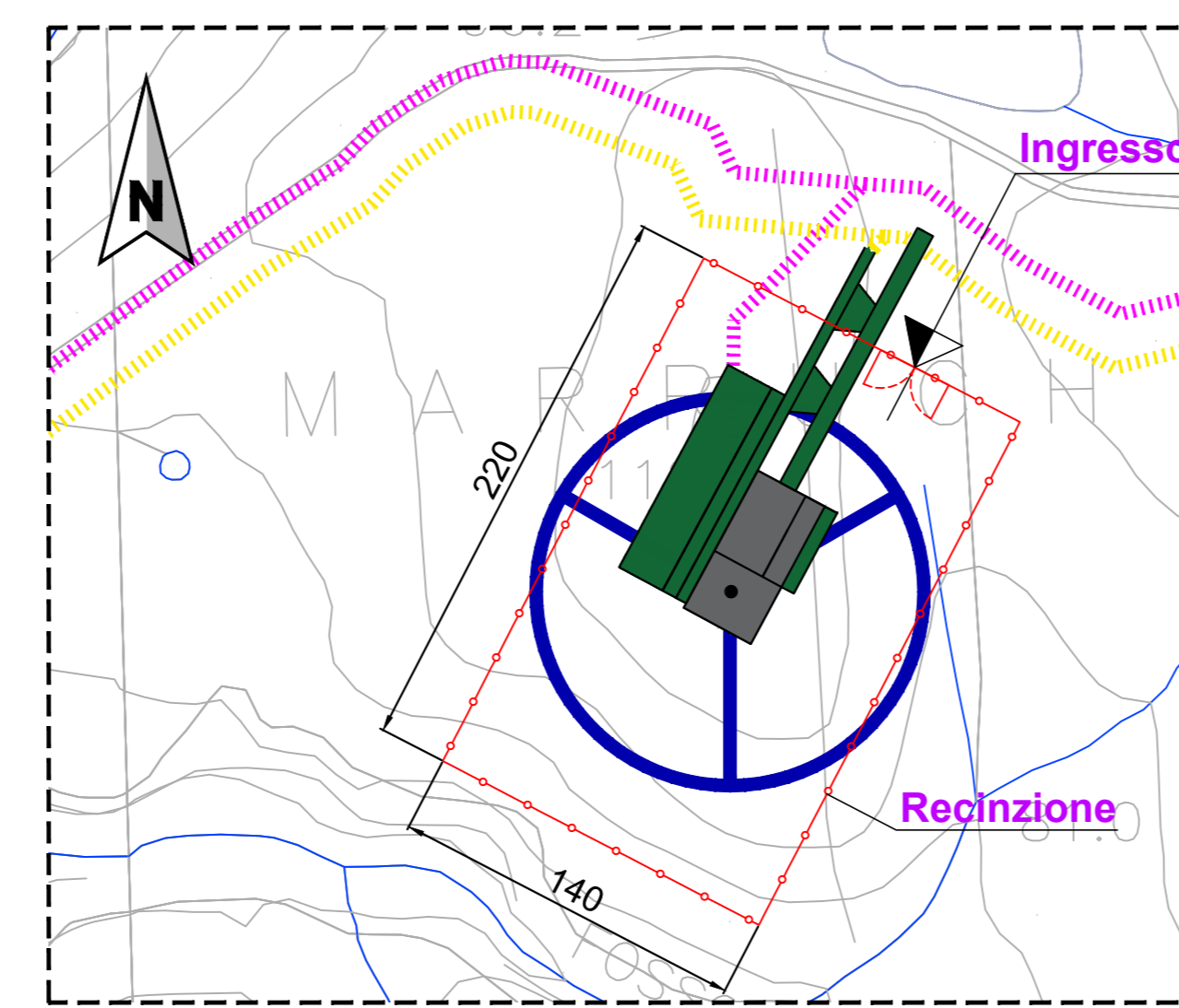
INQUADRAMENTO CANTIERE WTG5 (NON IN SCALA)
