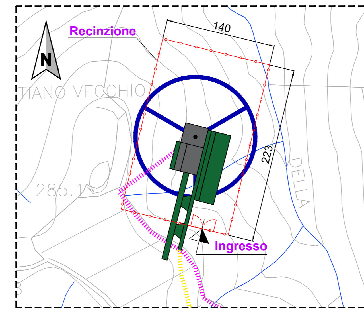
INQUADRAMENTO CANTIERE WTG11 (NON IN SCALA)
