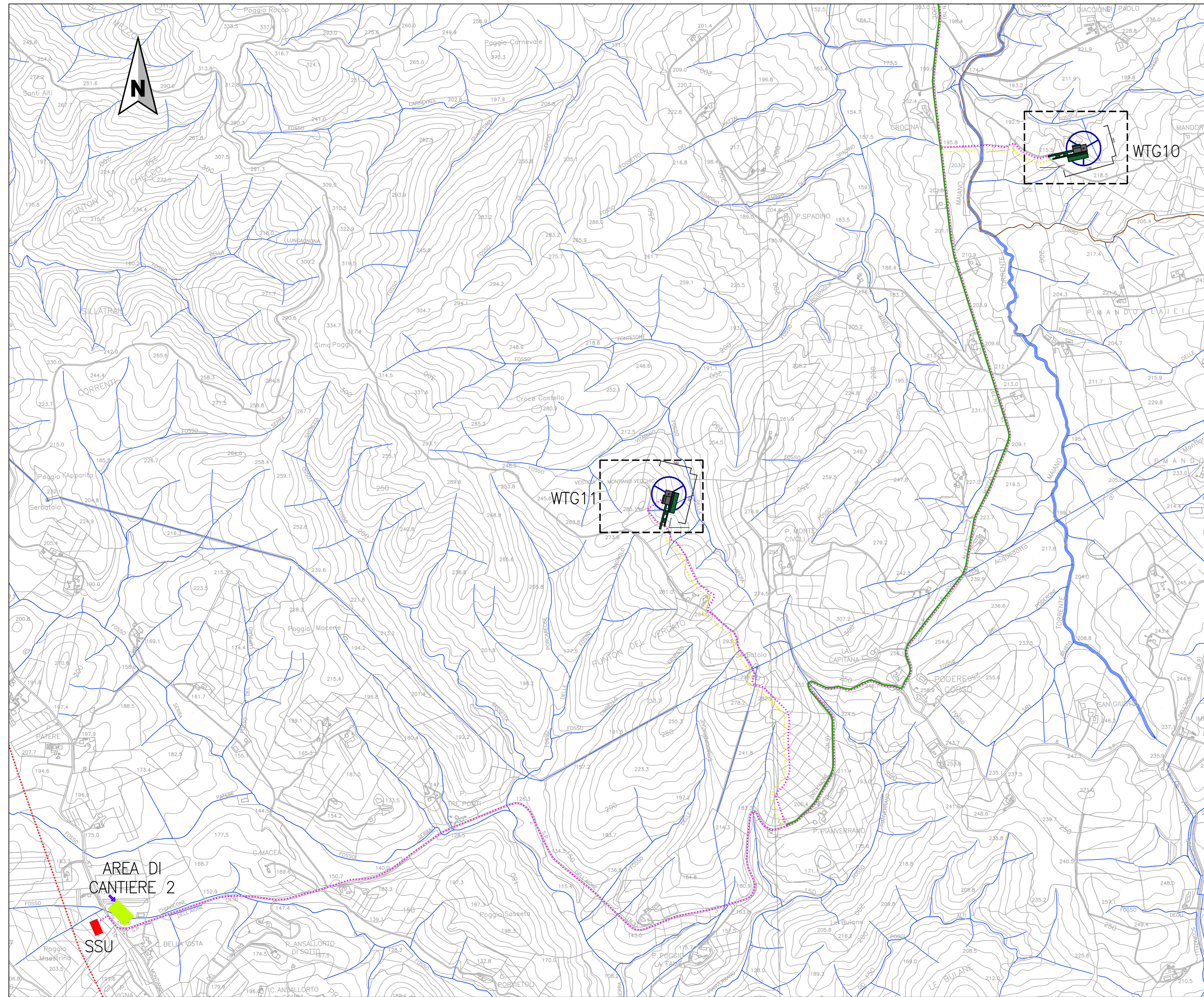
ESTRATTO PLANIMETRICO Scala 1:10000
