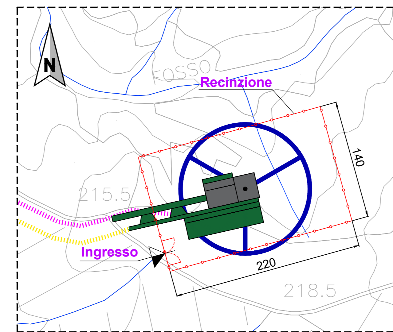
INQUADRAMENTO CANTIERE WTG10 (NON IN SCALA)
