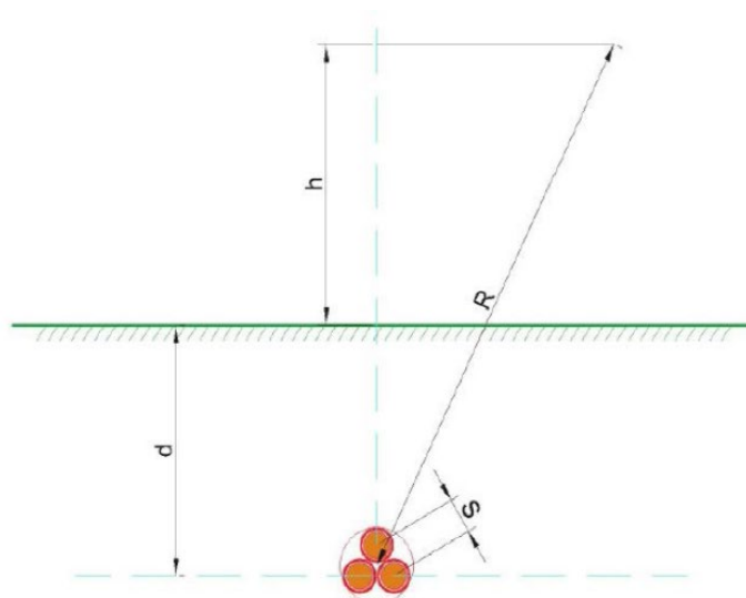
Geometria e disposizione spaziale della terna di vettoriamento
