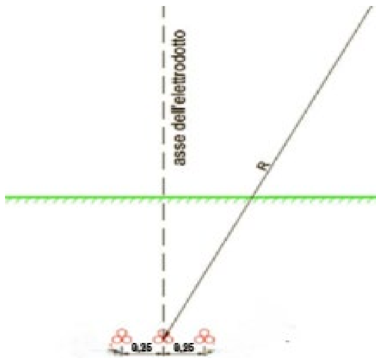
Geometria e disposizione spaziale delle terne di vettoriamento
