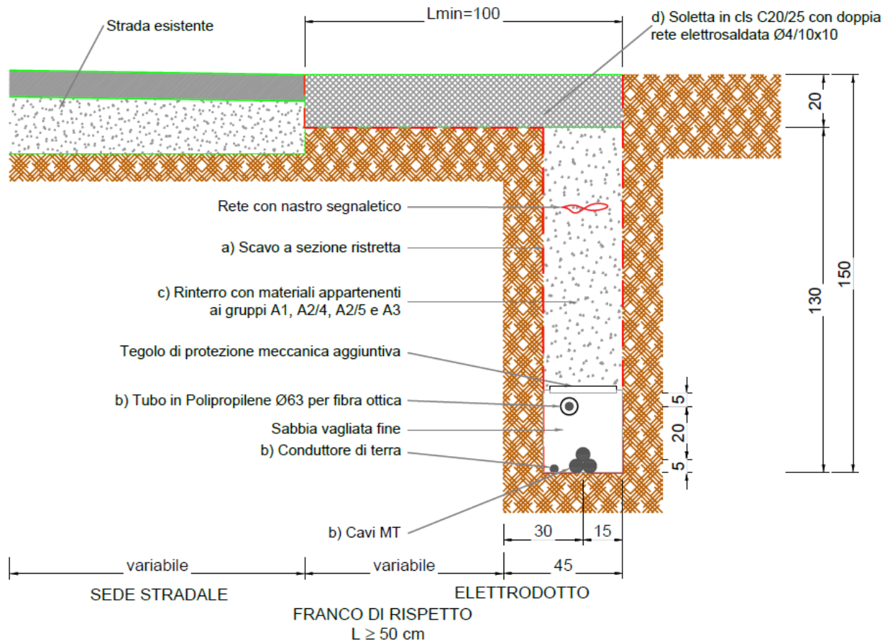
Tipologia di posa per cavidotto di vettoriamento MT in banchina di strada esistente in conglomerato bituminoso
