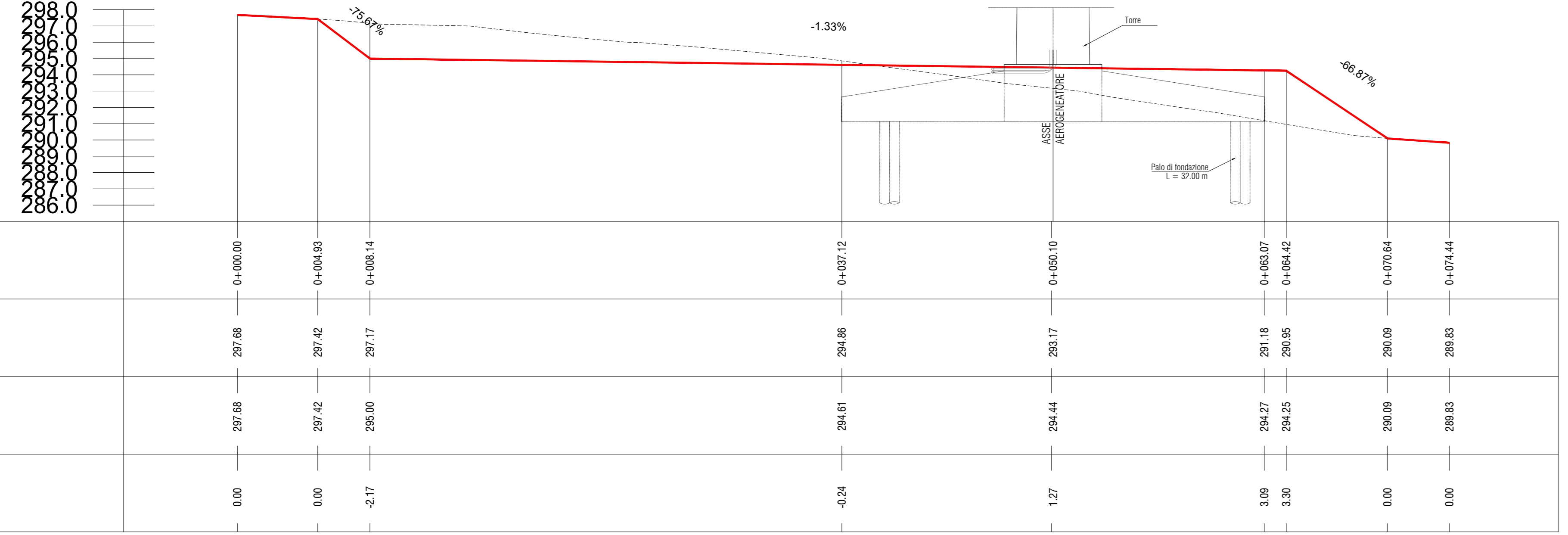
Profilo: Sezione A Scala: 1000:1000 Q.Rif.: 285.00
