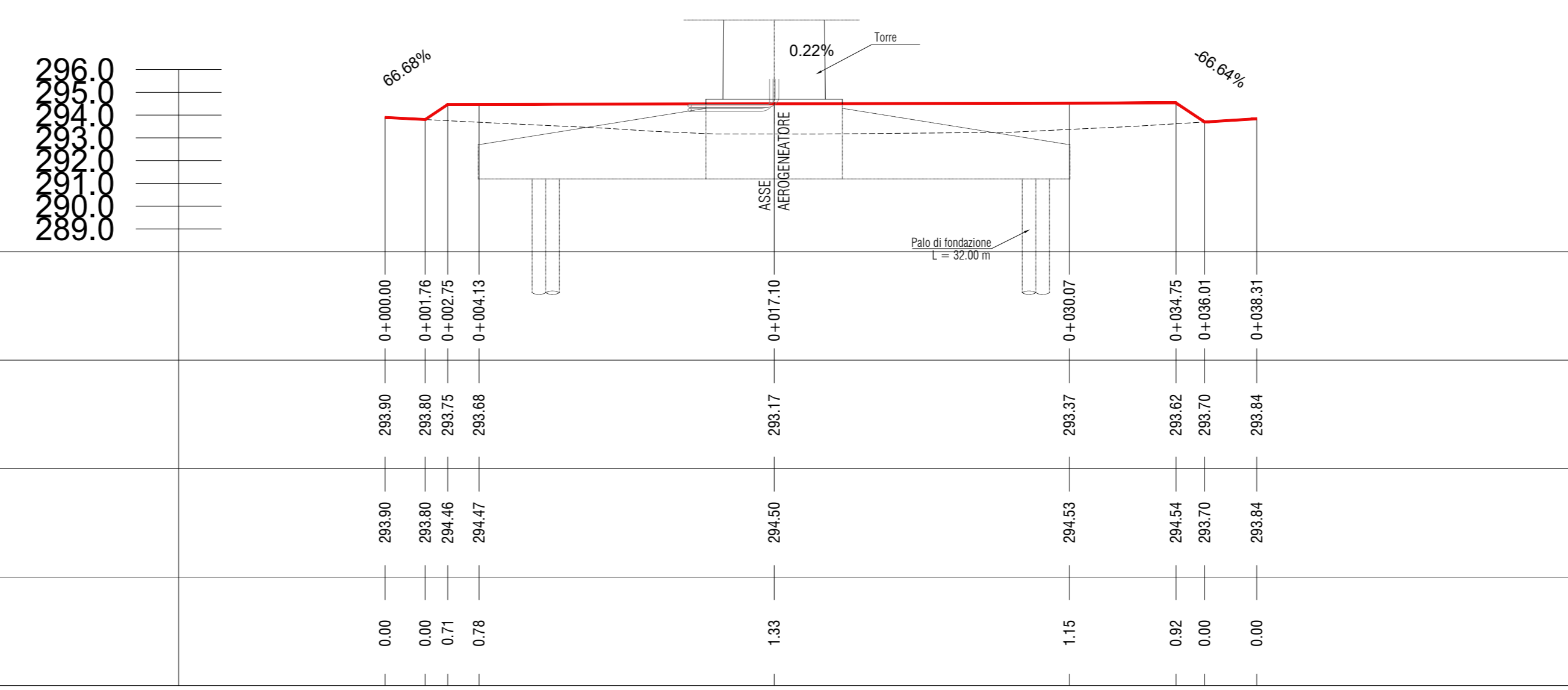
Profilo: Sezione B Scala: 1000:1000 Q.Rif.: 288.00
