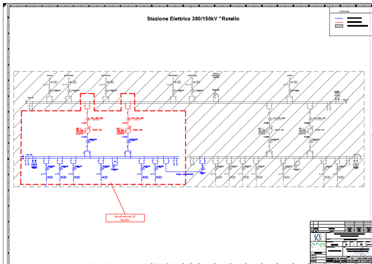
Figura 8 - Schema elettrico Generale + ampliamento della SE Rotello
