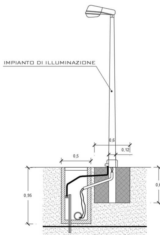
Fig. 23 – Sistema di illuminazione
