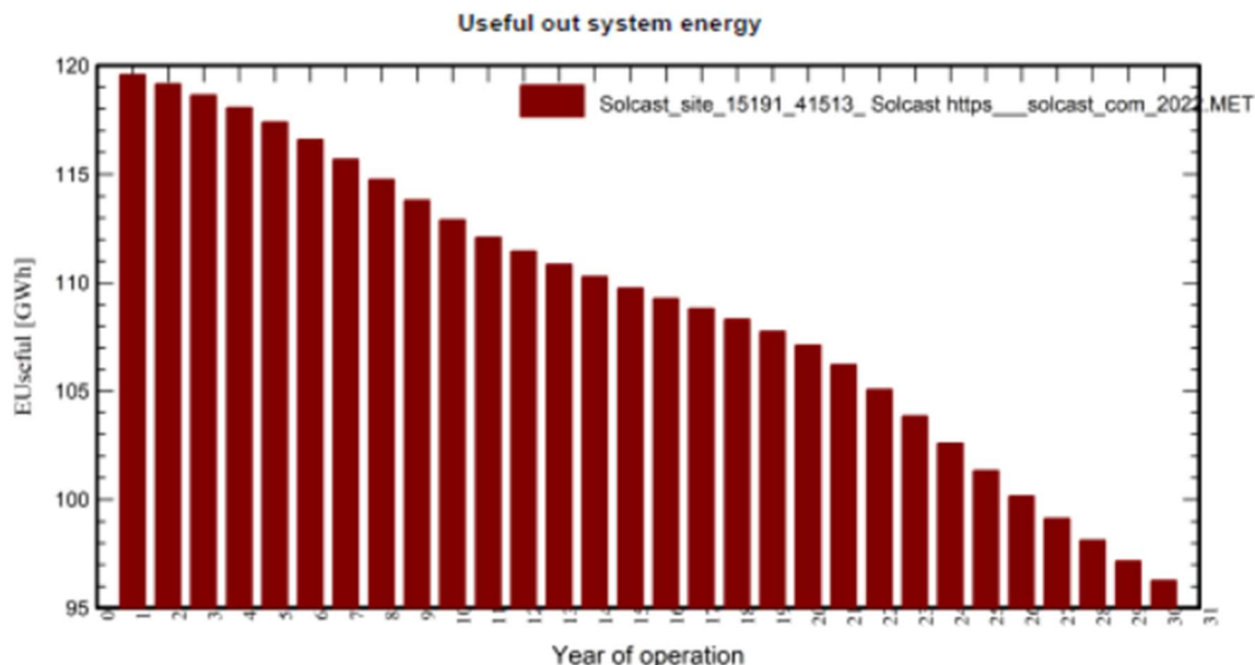
Fig. 28 – Producibilità dell’impianto con degrado moduli (30 anni)
