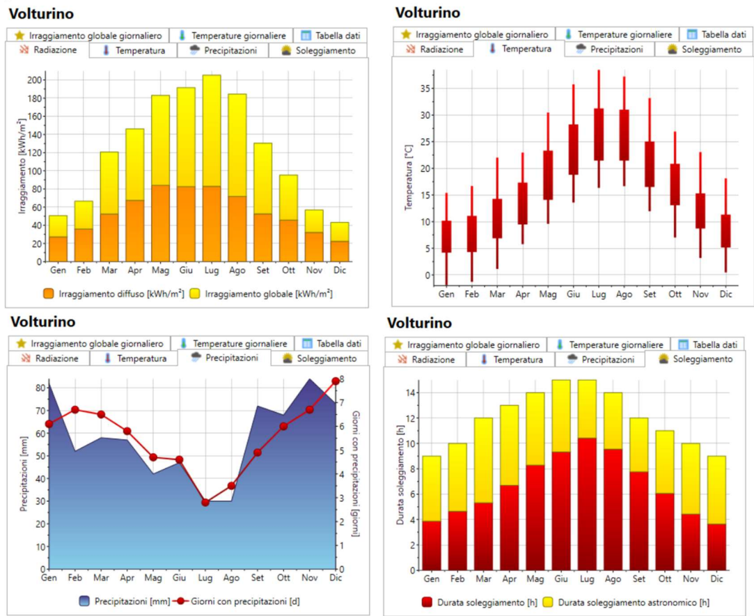
Fig. 24 – Dati di radiazione, temperatura, precipitazioni e soleggiamento
