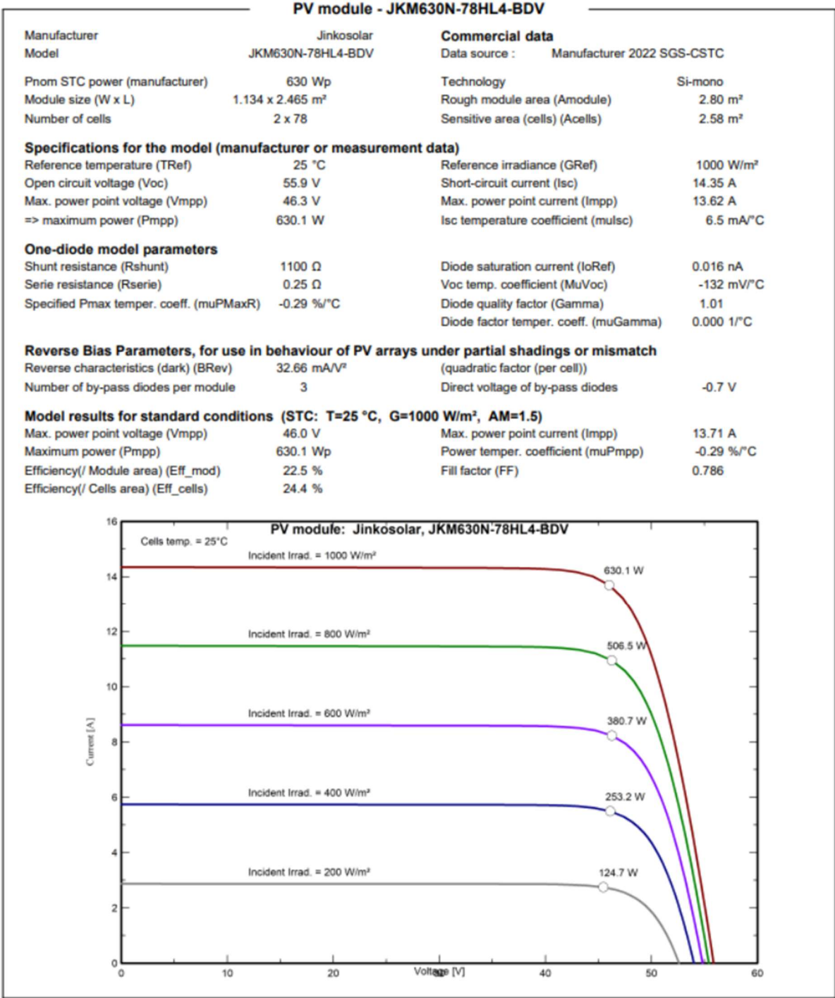
Figura 7 - Dimensioni, specifiche tecniche e prestazionali pannelli fotovoltaici Jinko Solar
