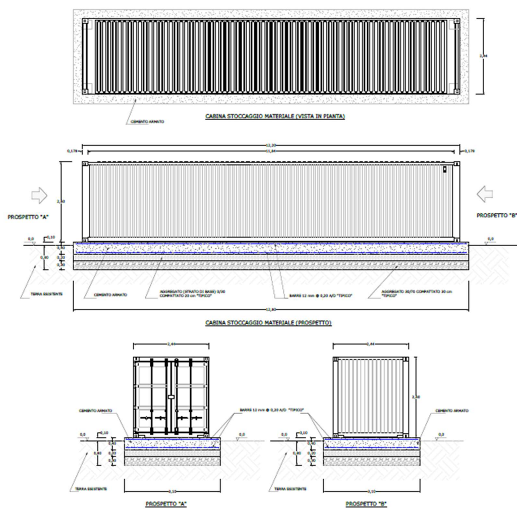
Fig. 21 - Cabina stoccaggio materiale
