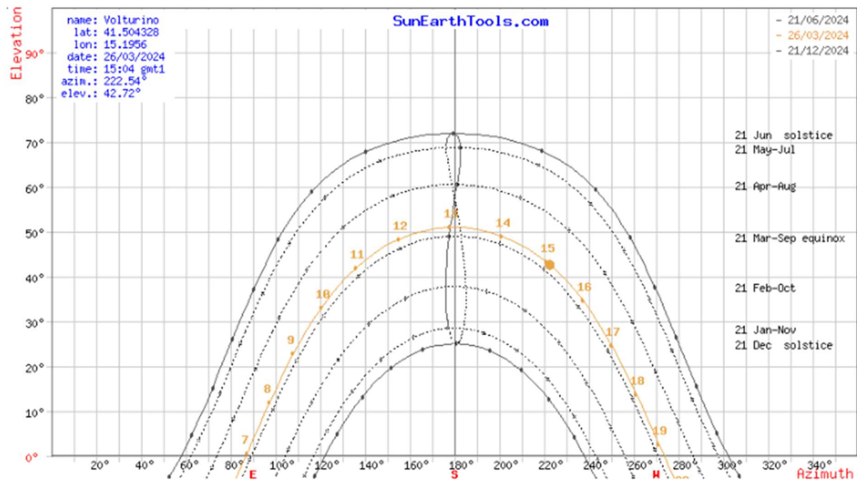
Fig. 26 - Diagramma Solare Polare (Volturino 63.3)
