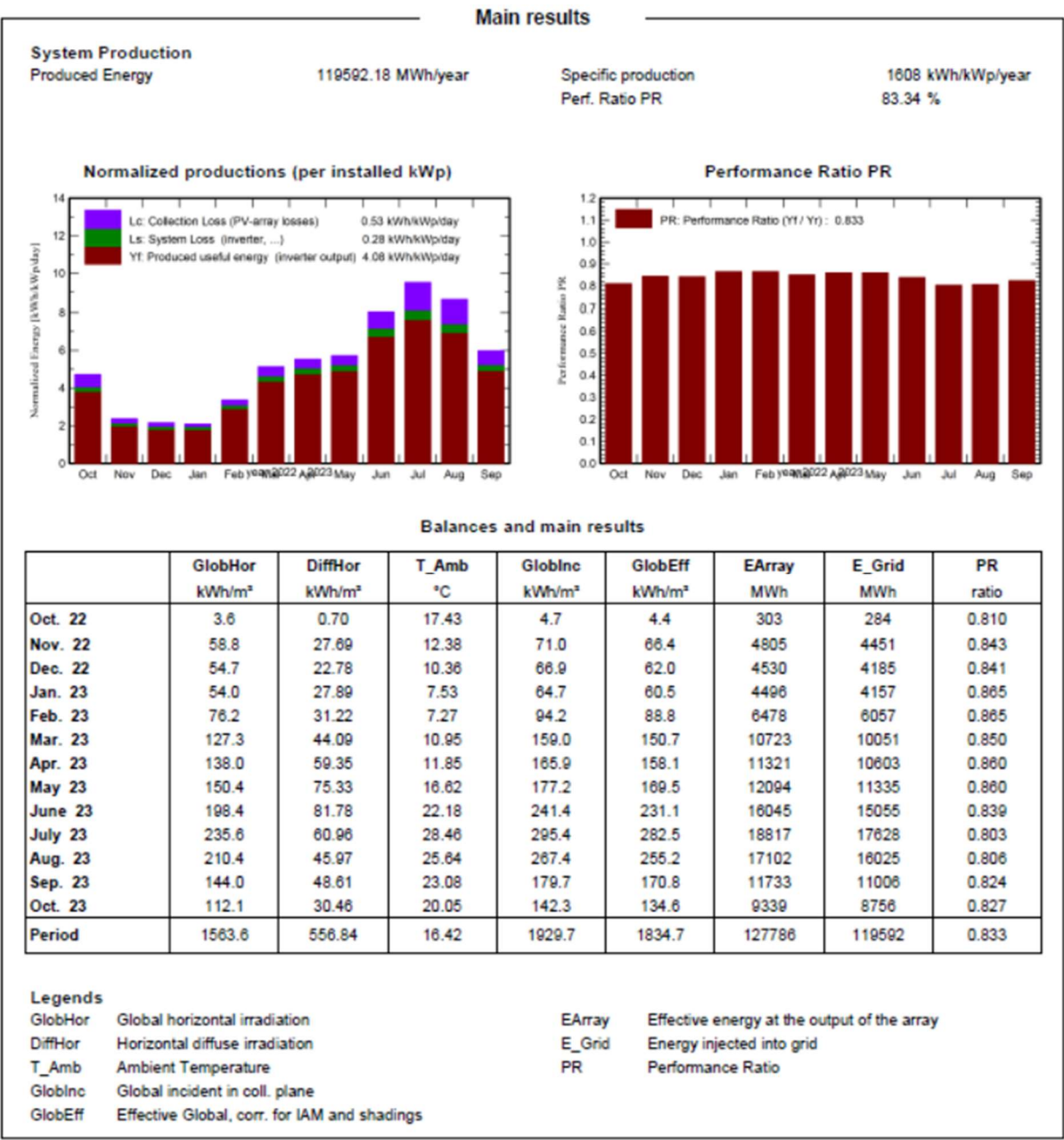
Fig. 27 - Risultati di calcolo (Fonte: PVsyst - Meteonorm)
