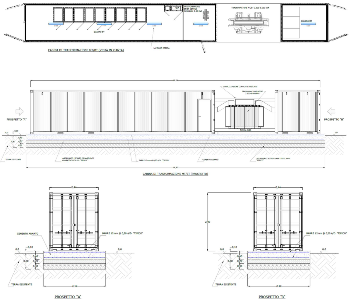
Fig. 18 - Cabina di trasformazione MT/BT
