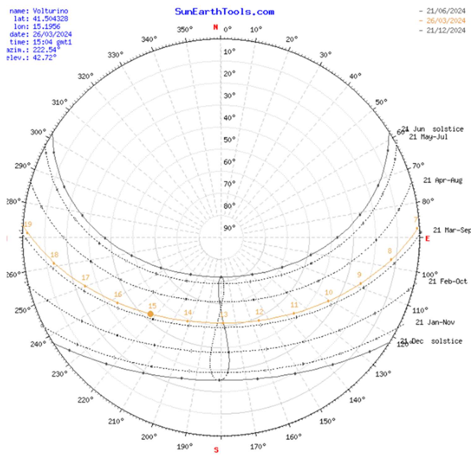
Fig. 25 - Diagramma Solare Polare (Volturino 63.3)
