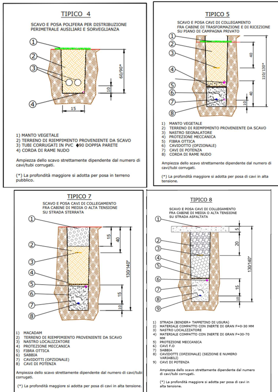
Fig. 17 – Tipici scavi e posa cavi
