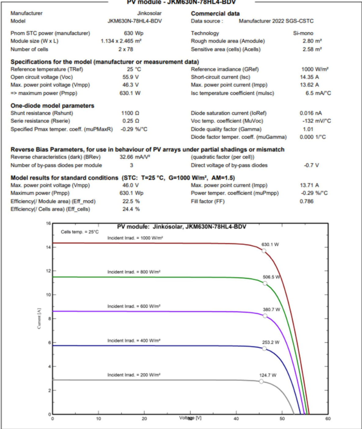
Fig. 1 - Dimensioni, specifiche tecniche e prestazionali pannelli fotovoltaici Jinko Solar
