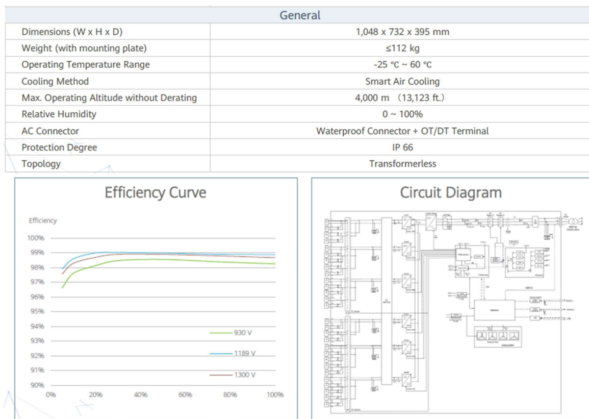
Fig. 6 - Dimensioni, specifiche tecniche e prestazionali dell'inverter
