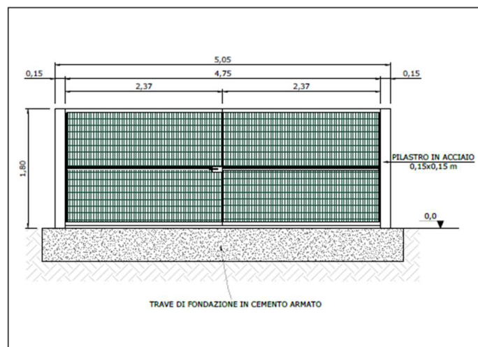
Fig. 16 – Cancello carrabile
