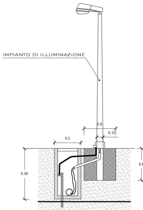
Fig. 19 – Sistema di illuminazione
