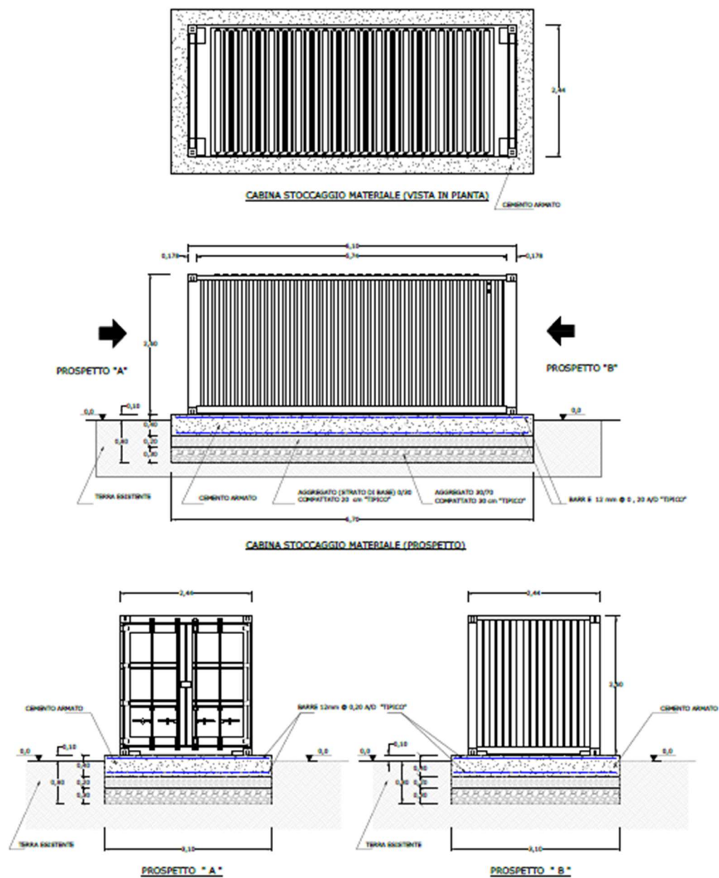
Fig. 13 - Cabina stoccaggio materiale
