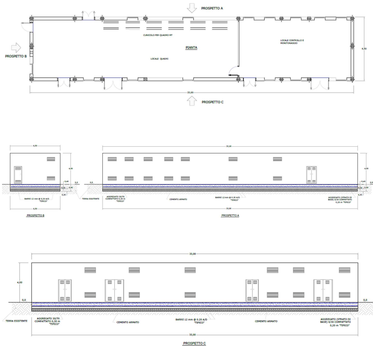
Fig. 12 - Cabina di ricezione, sezionamento e controllo
