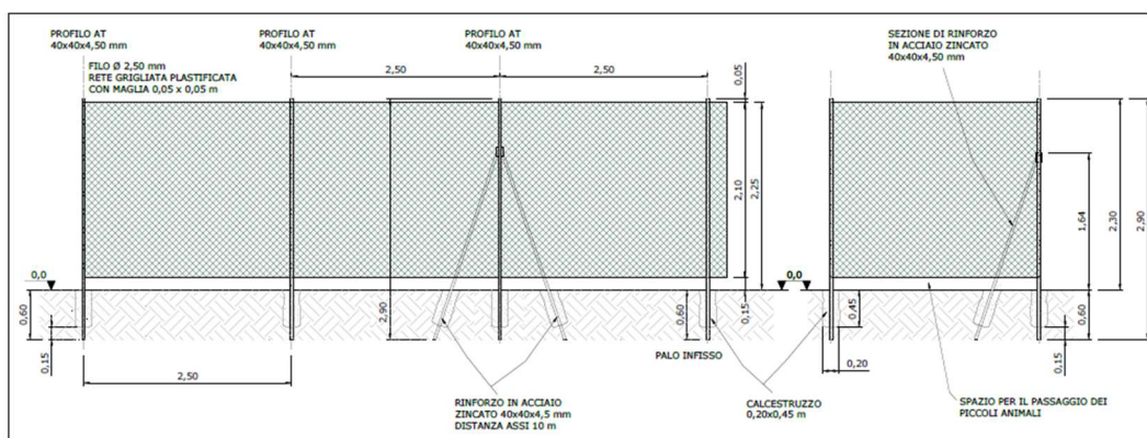
Fig. 15 – Particolare della recinzione
