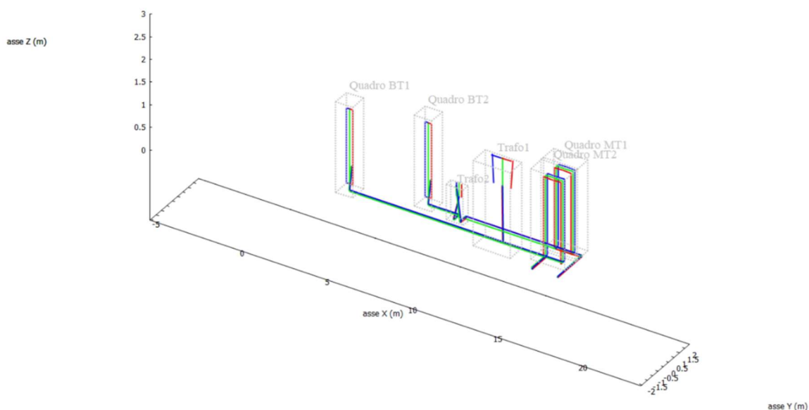
Fig.6 - Modello spaziale cablaggi nelle cabine di trasformazione MT/BT
