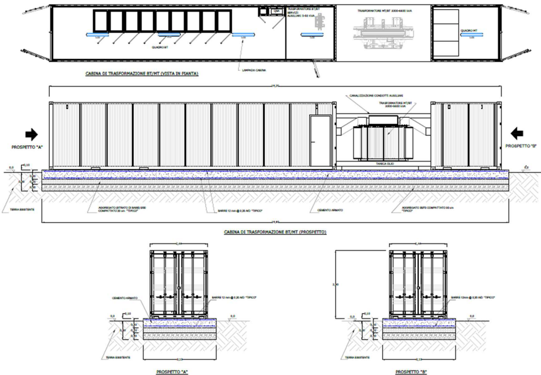
Fig.4 - Ingombri cabine di trasformazione MT/BT
