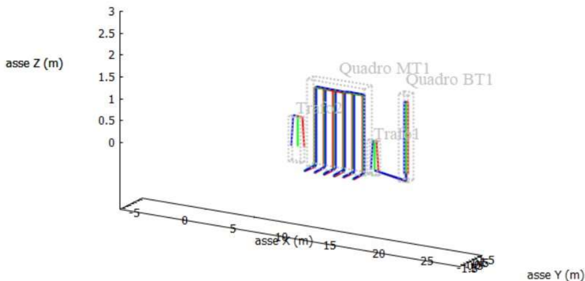
Fig.7 - Modello spaziale cablaggi nelle cabine di ricezione
