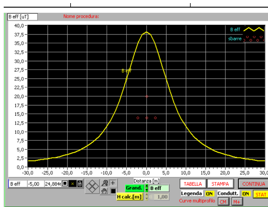
Fig. 13: Andamento campo magnetico
