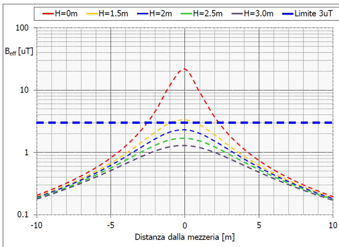
Fig. 8: Andamento dell'induzione magnetica prodotta dalla linea in cavo per la massima corrente del cavo
