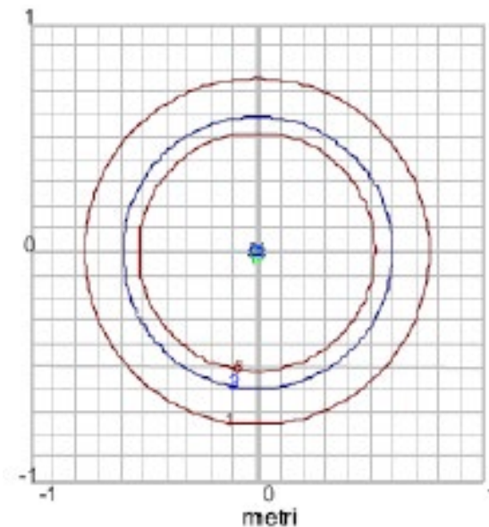
Fig. 6: Curve di equilivello per il campo magnetico di una linea MT in cavo elicordato interrata (dalla Norma CEI 106-11)
