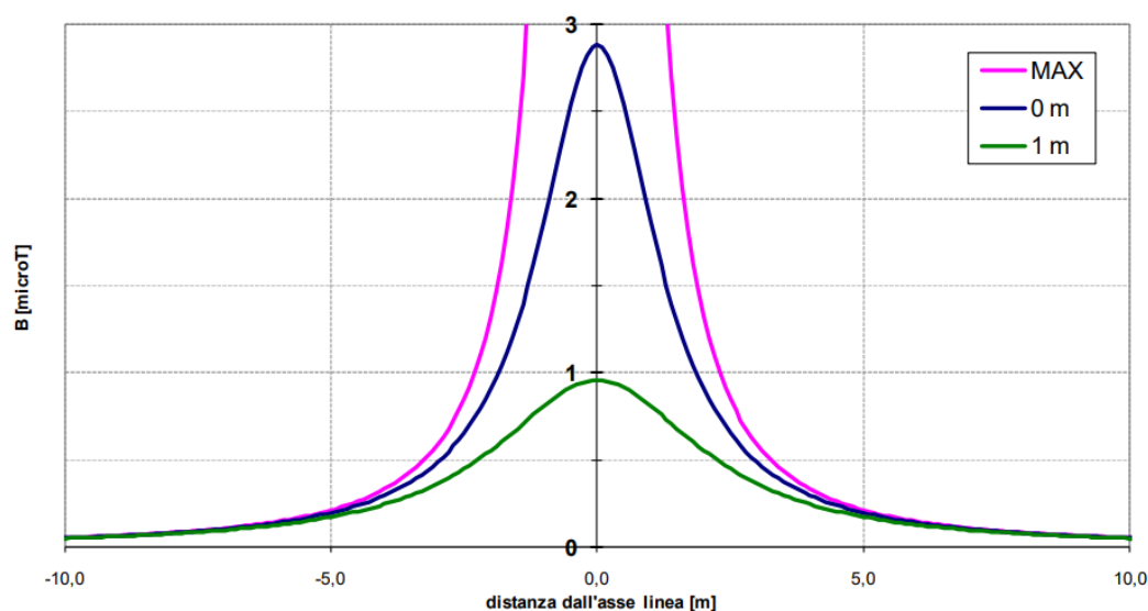
Fig. 14: Andamento dell'Induzione magnetica prodotta dalla linea in cavo
