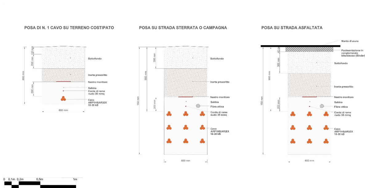
Fig.7: Sezione tipica di posa della linea in cavo
