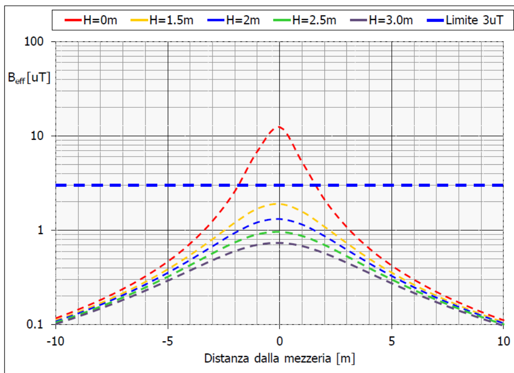
Fig. 9 - Andamento dell'induzione magnetica prodotta dalla linea in cavo per la massima corrente dell'impianto
