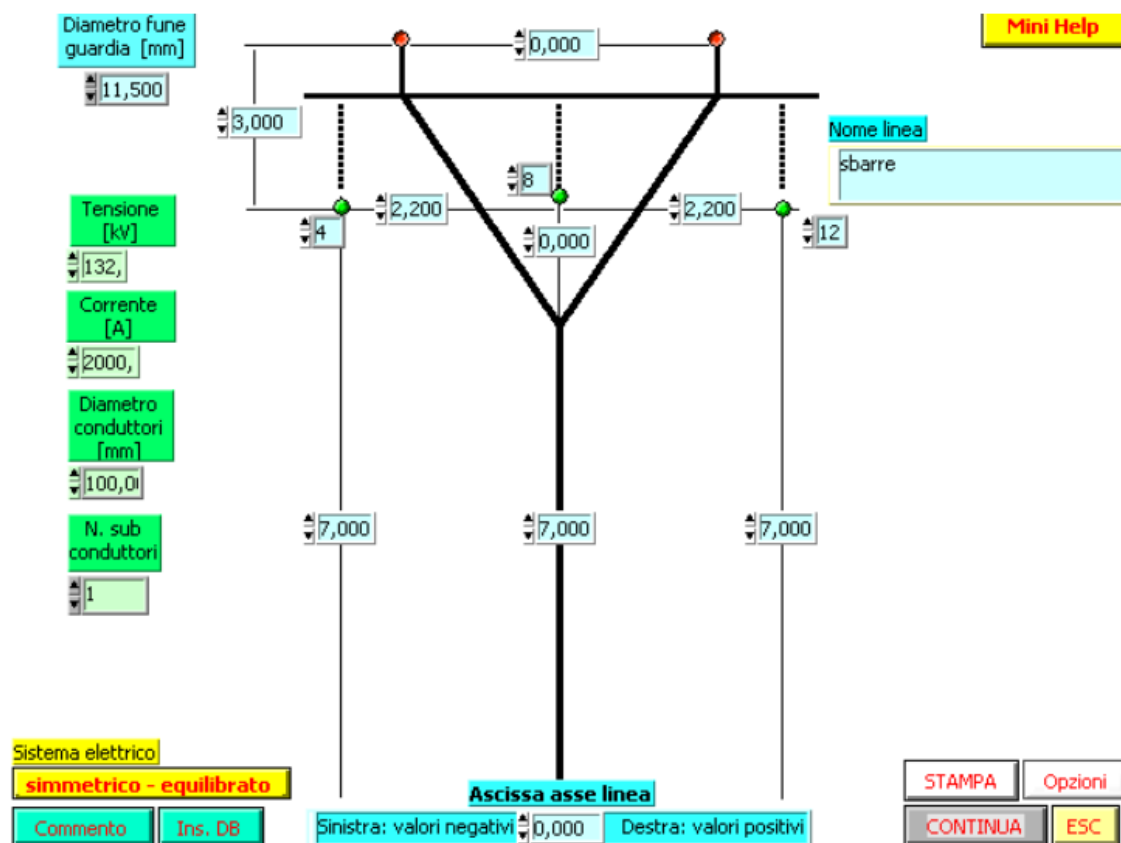
Fig. 12: Geometria "tipo" di un sistema trifase
