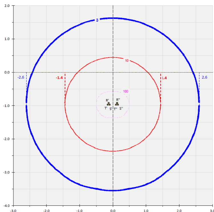
Fig. 10 - Curve di equilivello per il campo di induzione magnetica generato da una linea MT posata a trifoglio ( I_{\max}=725 A; formazione 3x1x630)
