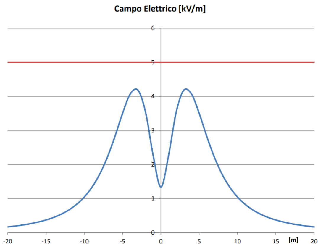
Fig. 11: Campo elettrico al suolo generato dal sistema di sbarre a 220 kV
