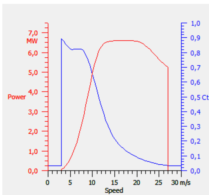
Figura I - Curva di potenza e Ct dell'aerogeneratore Siemens-Gamesa SG155 6,6MW
