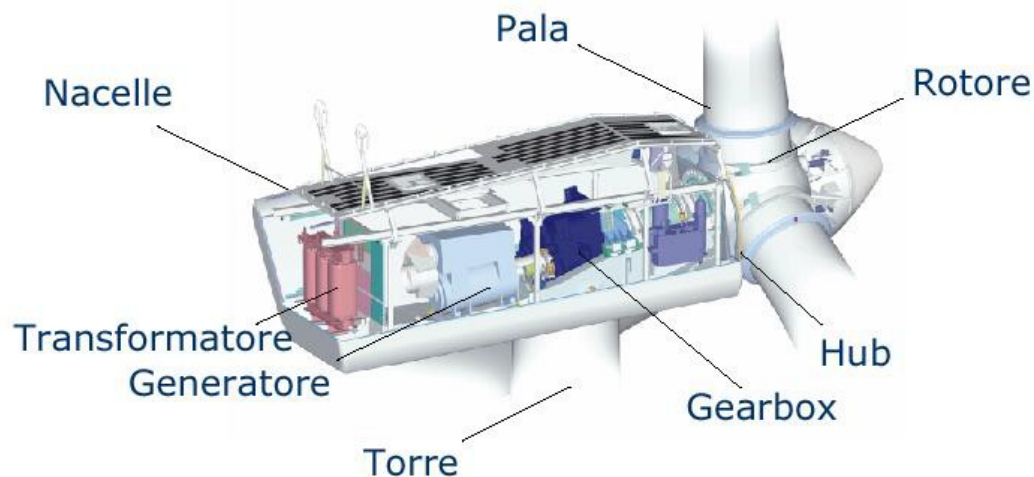
Figura 1 – Elementi dell'aerogeneratore
