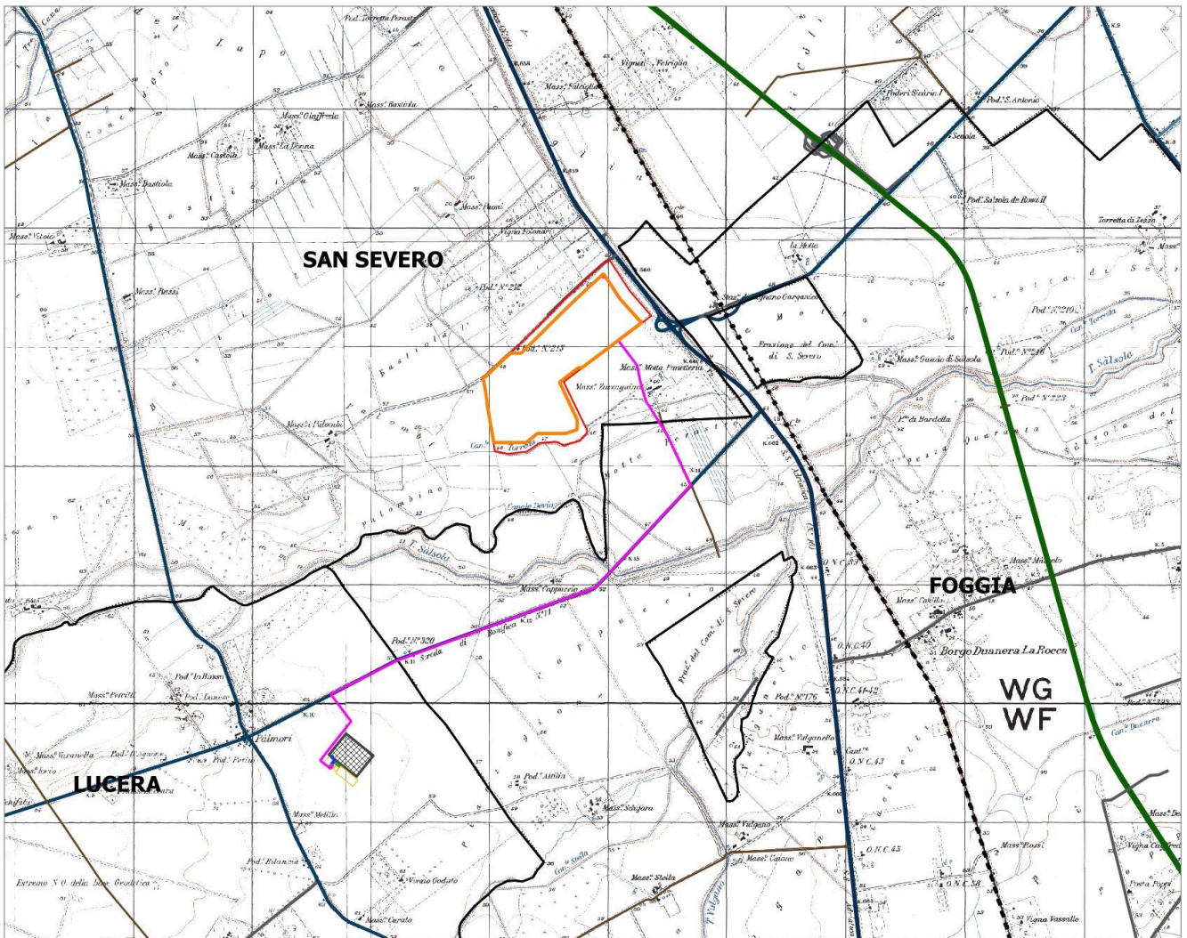
Figura 4 - Tracciato cavidotto MT su base IGM
