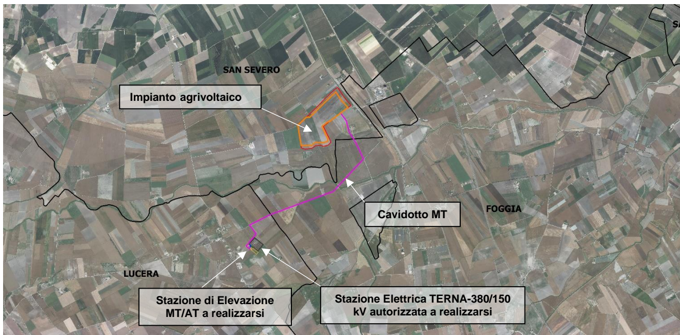
Figura 1 - Inquadramento su base ortofoto area impianto agrivoltaico “San Severo” e futura SE RTN 380/150 kV
