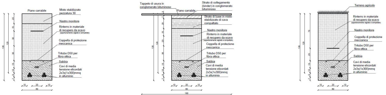
Figura 3 - Particolari sezioni cavidotto esterno MT su strada asfaltata, non asfaltata e terreno agricolo
