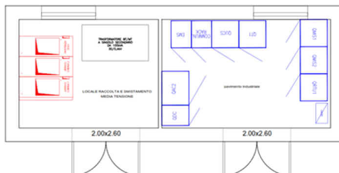
Figura 13 – Tipico Cabina di raccolta e smistamento
