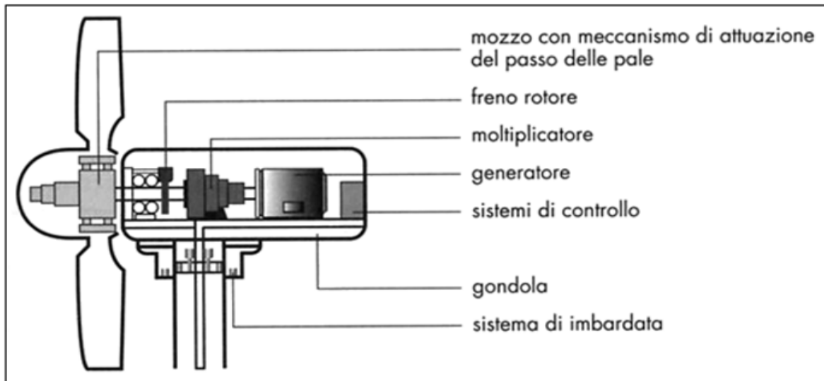
Figura 6: Schema di principio di un aerogeneratore
