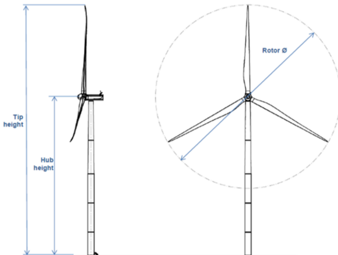
Figura 5: Esempio aerogeneratore
