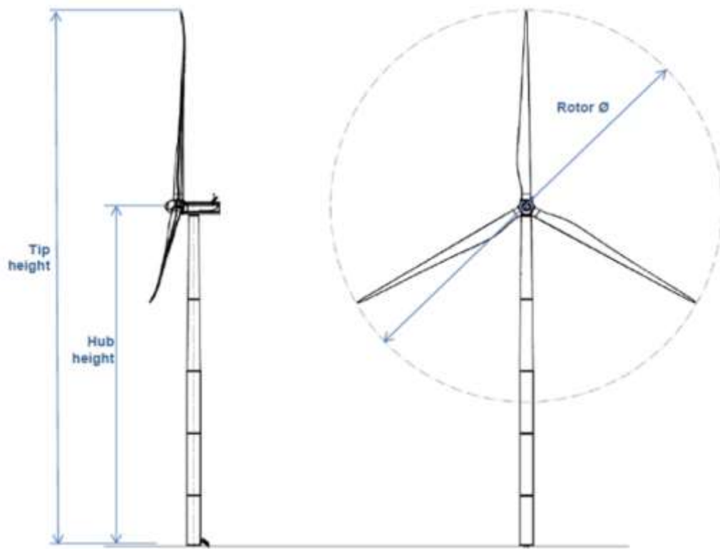
Figura 3: Esempio Aerogeneratore
