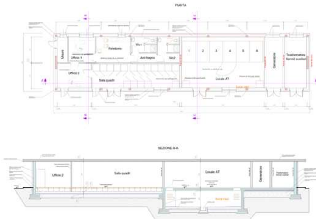
Figura 12: Planimetria e sezioni della SSE di raccolta e controllo
