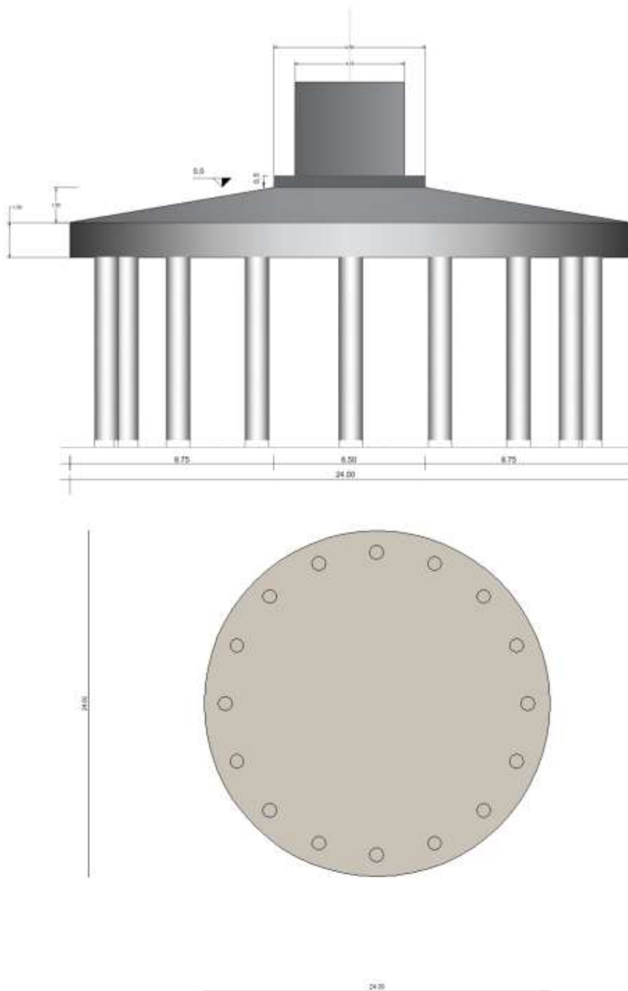
Figura 5: Pianta e schema geometrico tipo
