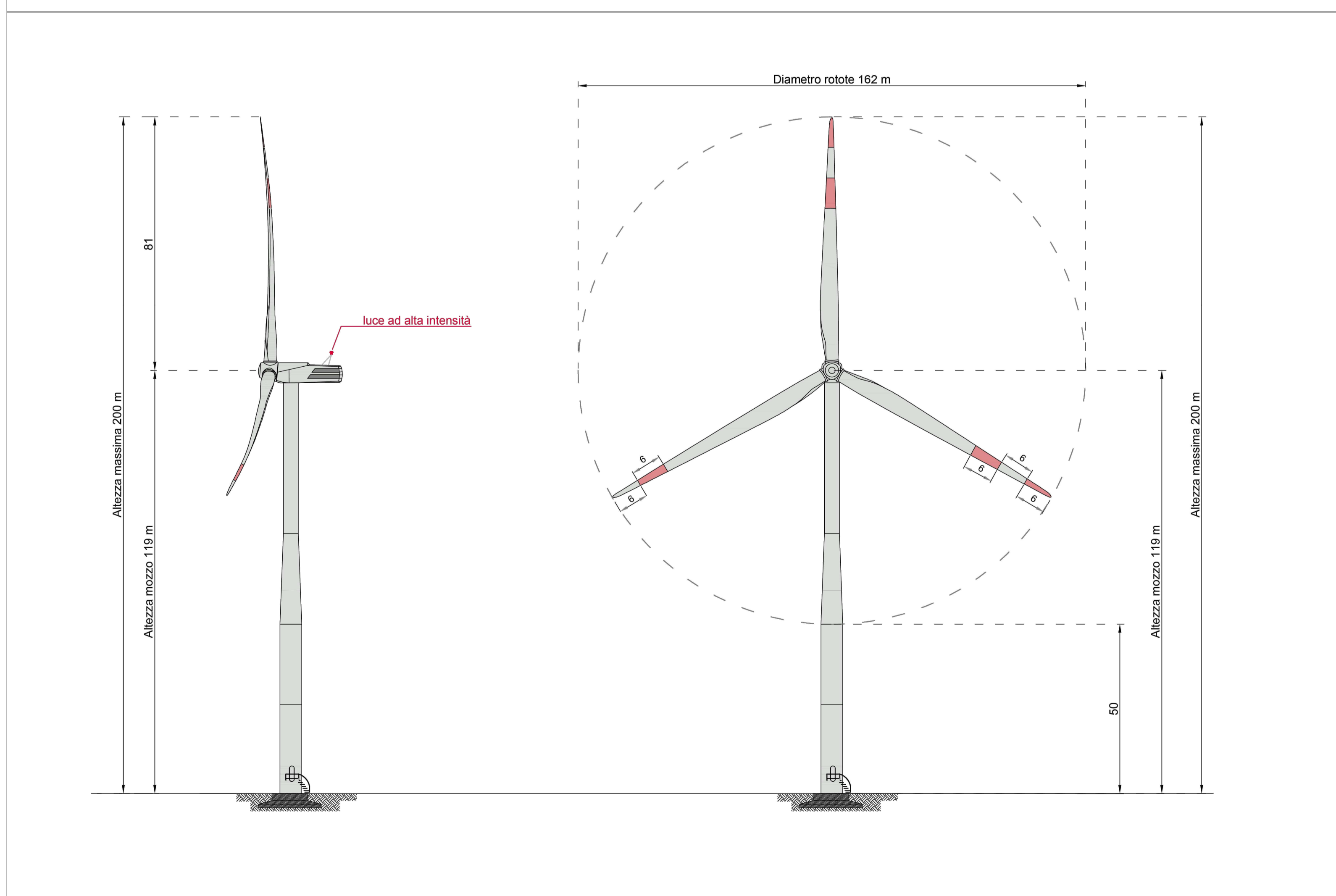
Viste prospettiche Aereogeneratore tipo
