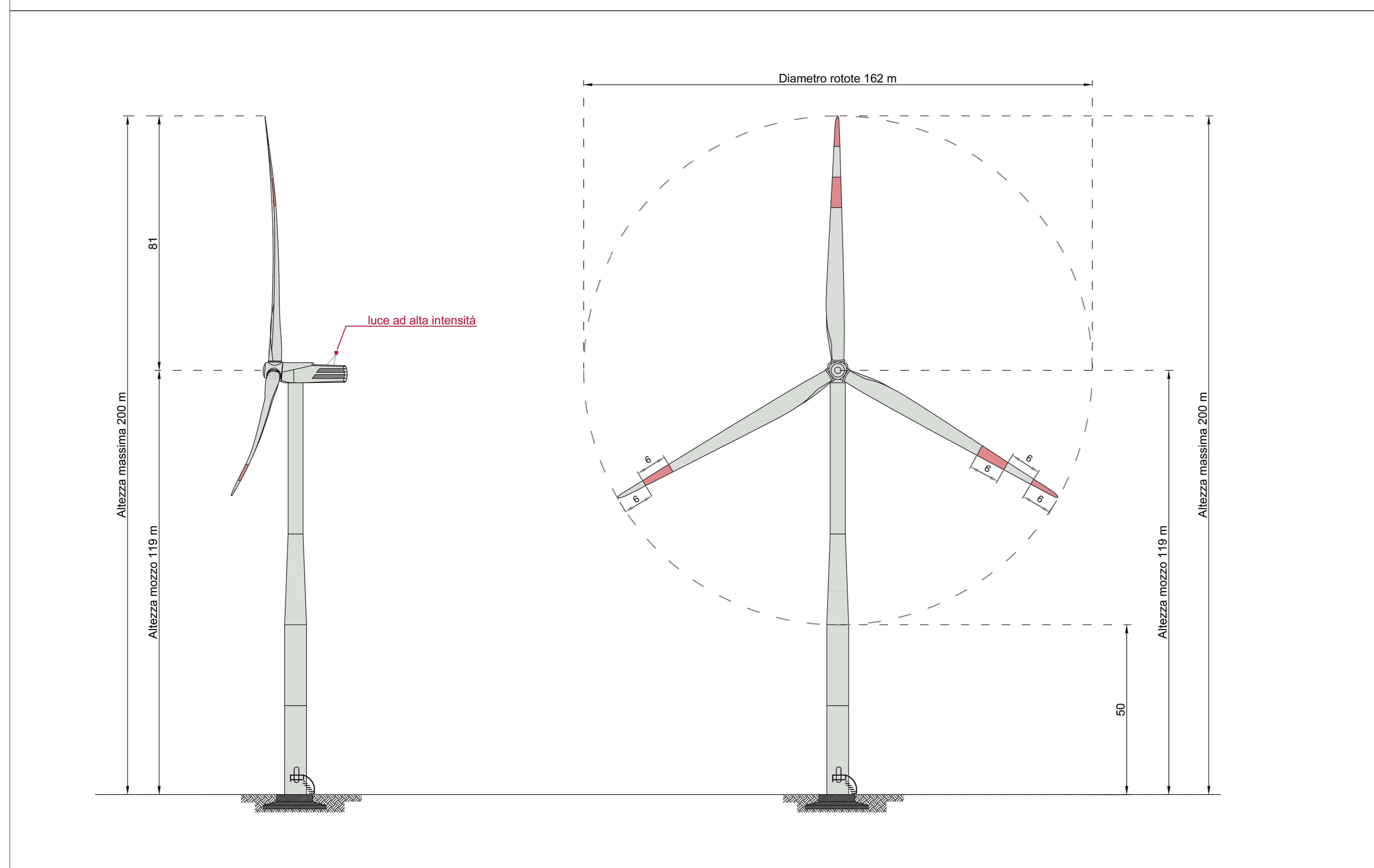
Viste prospettiche Aereogeneratore tipo
