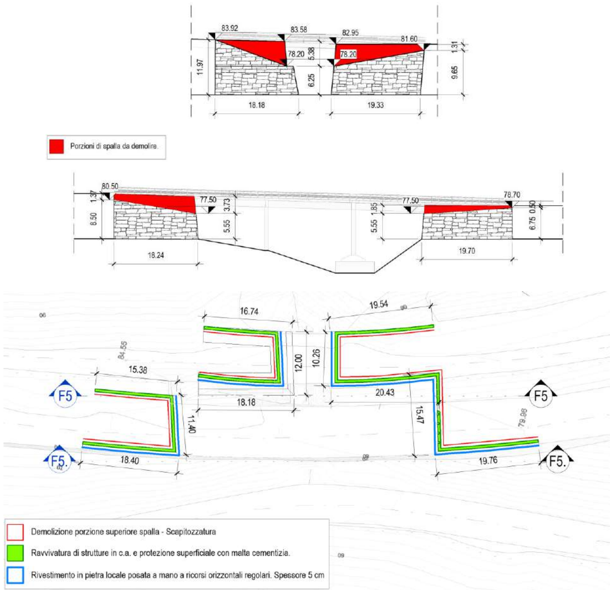
Figura 6.1: Individuazione aree da demolire Spalle e rivestimento in pietra
