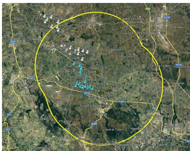
Figura 2 – Individuazione degli aerogeneratori di progetto su cartografia rispetto alla presenza di impianti eolici autorizzati e/o in fase di autorizzazione
