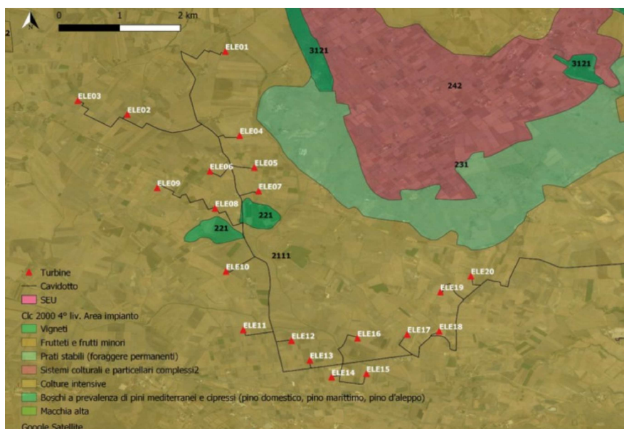
Figura 7 – Carta uso del suolo – CLC
