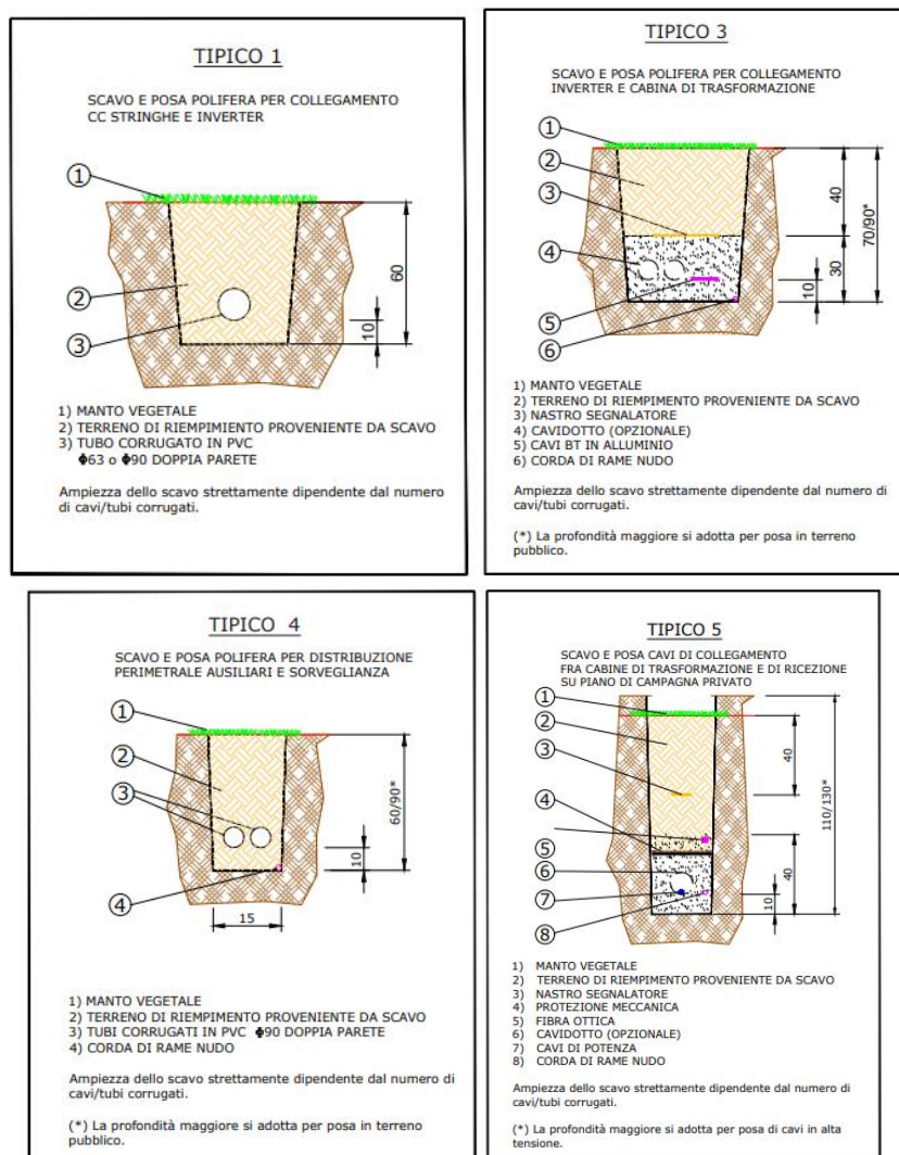
Fig. 6 – Tipici scavi e posa cavi
