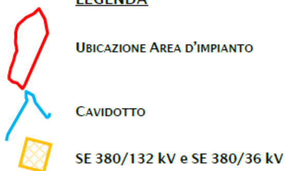
Fig. 5 – Stralcio della carta idrogeologica e delle aree con problematiche idrogeologiche – TAV. 6.e.7 (AI SENSI DEL DPGRT 26/R/07)
