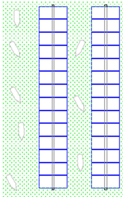
Fig. 2 – Piantumazione tra le file di tracker (vista dall'alto)
