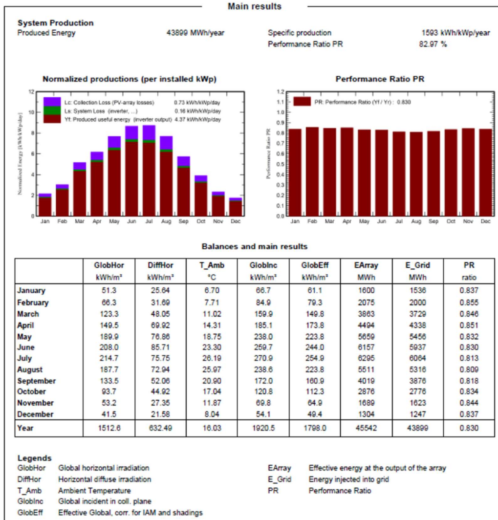
Fig. 26 - Risultati di calcolo (Fonte: PVsyst - Meteonorm)
