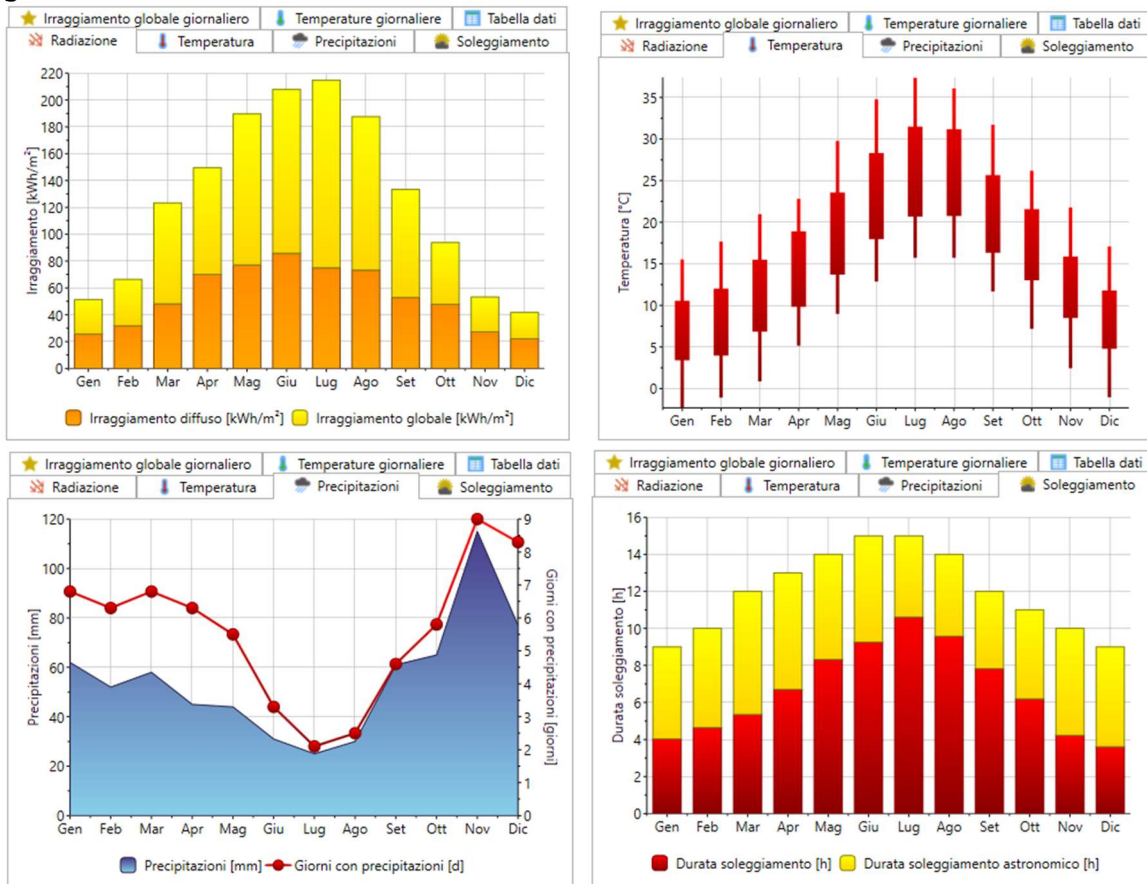
Fig. 23 – Dati di radiazione, temperatura, precipitazioni e soleggiamento (Riferiti al sito di Manciano)
