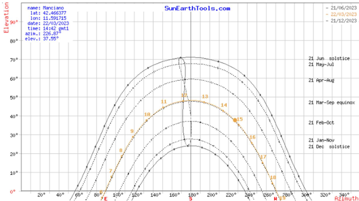
Fig. 25 - Diagramma Solare Polare (Manciano)
