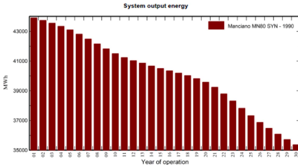
Fig. 27 – Producibilità dell’impianto con degrado moduli (30 anni)
