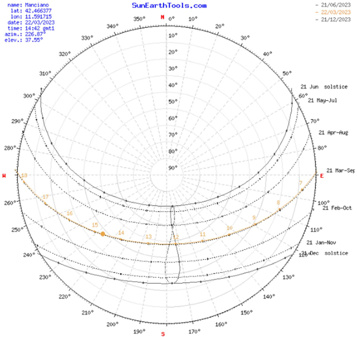
Fig. 24 - Diagramma Solare Polare (Manciano)
